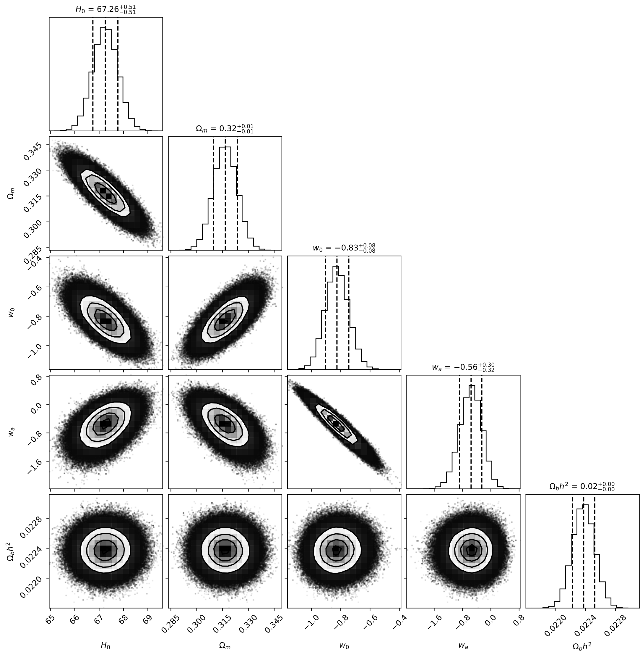
CPL posterior (N=25000, covarianza DESI completa)
