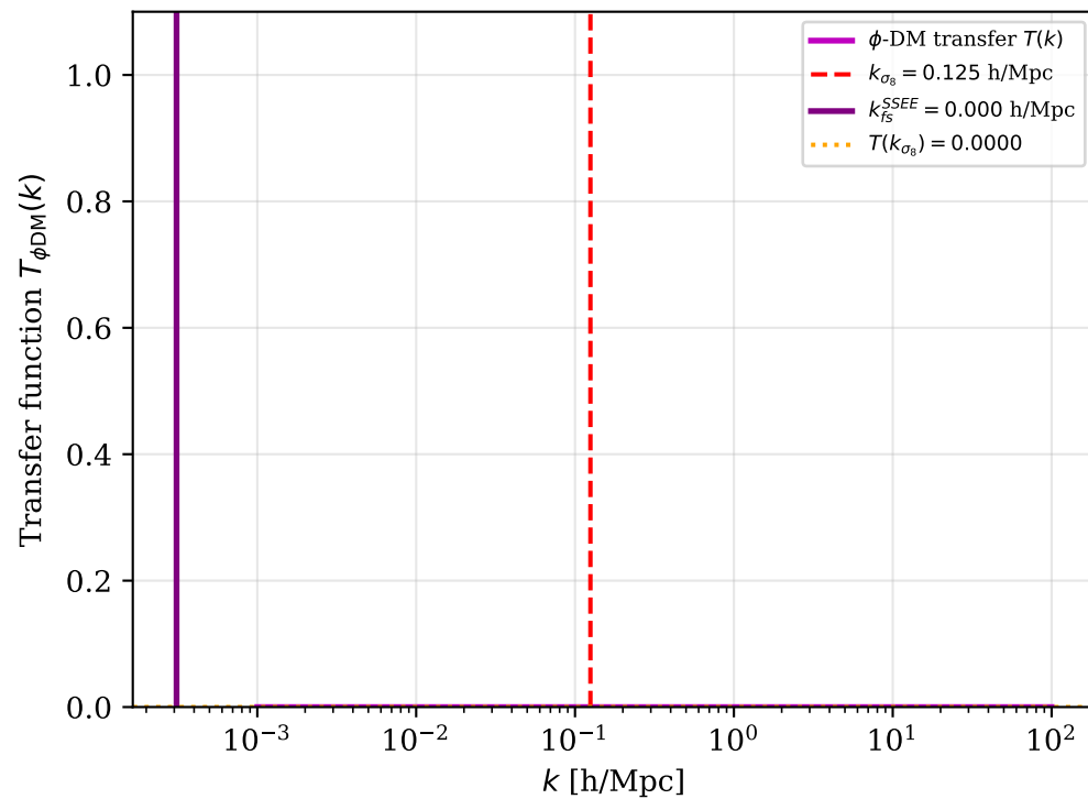
\phi -DM Suppression
