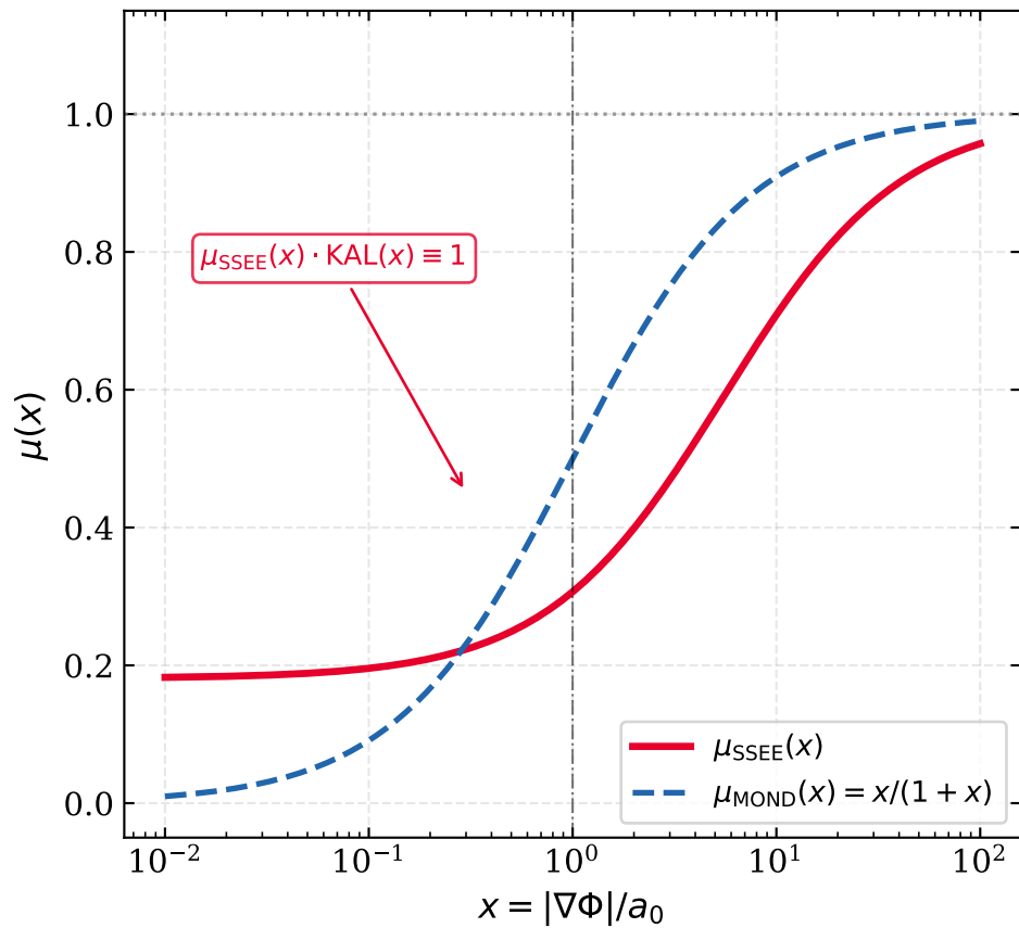
\mu_{SSEE} vs \mu_{MOND} — dualidad asimétrica
