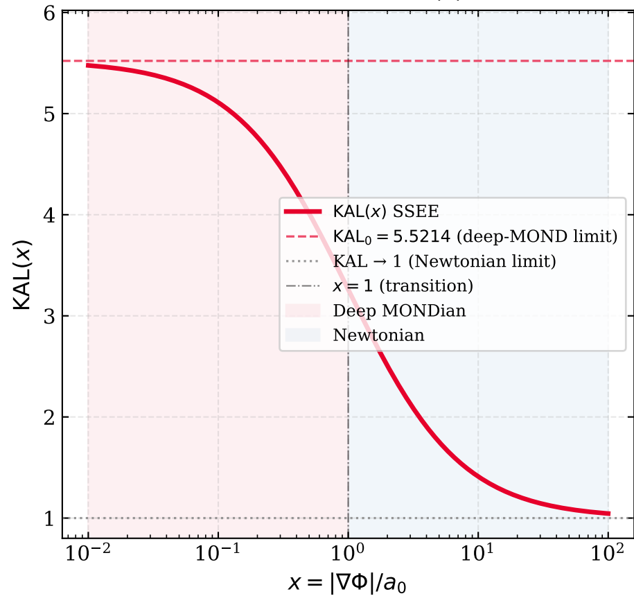
Viscosidad estructural KAL(x) - SSEE
