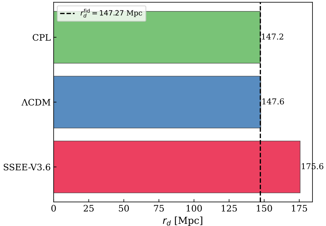
Horizonte de sonido r_d (MAP)
