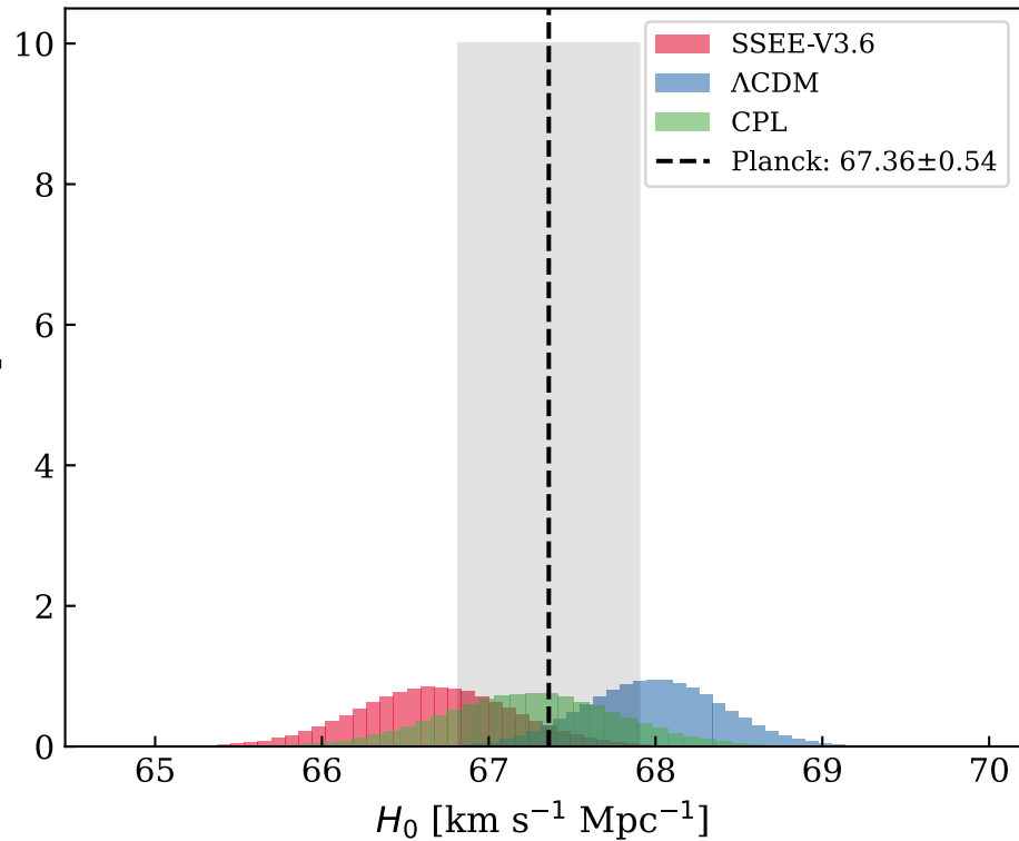
Posterior H_0 — comparación de modelos
