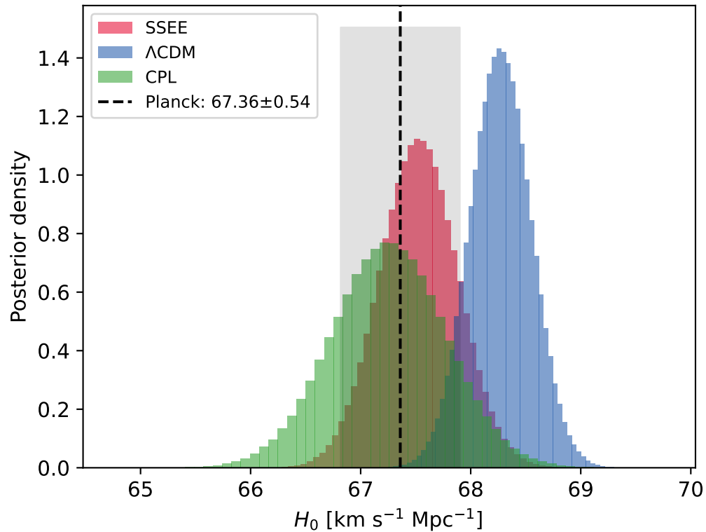
H_0 posteriors — SSEE 67.53 \pm 0.35 ( 0.26\sigma Planck)
