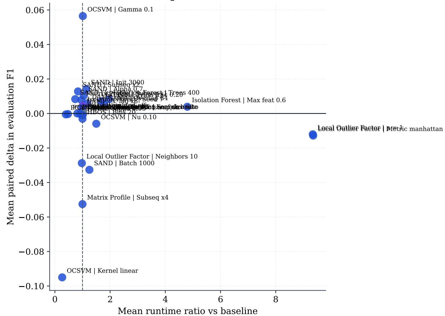
Runtime tradeoff vs paired evaluation F1 delta
