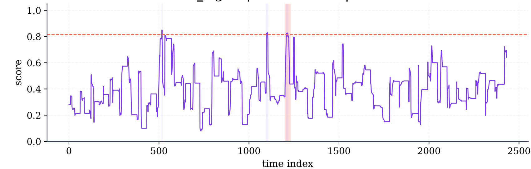
Variant 3: x_lag x8 | Eval F1=0.30 | ROC AUC=0.90
