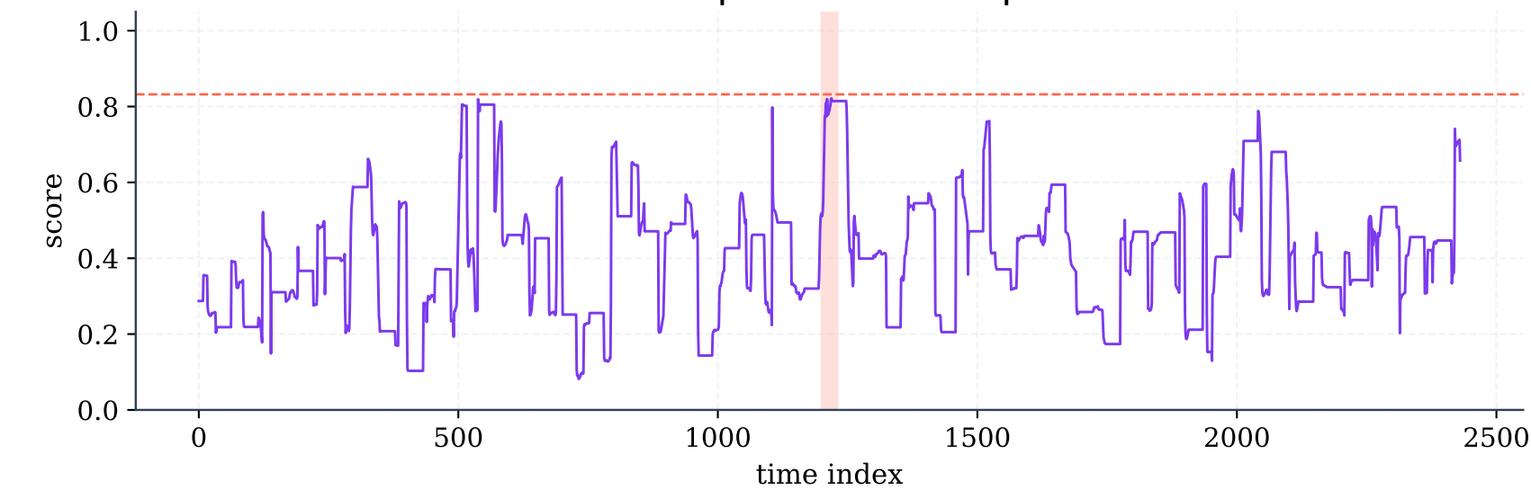
Variant 3: x_lag x8 | Eval F1=0.30 | ROC AUC=0.90
