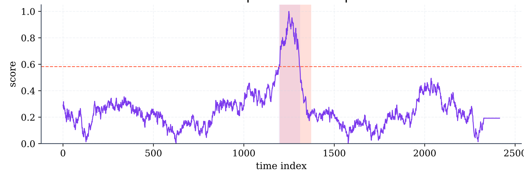
Variant 4: Max feat 0.6 | Eval F1=0.45 | ROC AUC=0.92
