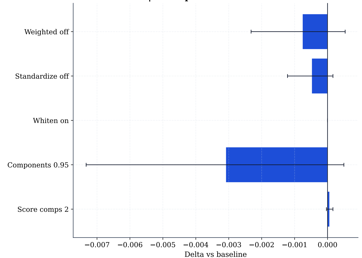
PCA | Mean paired delta in evaluation F1 by dataset variant
