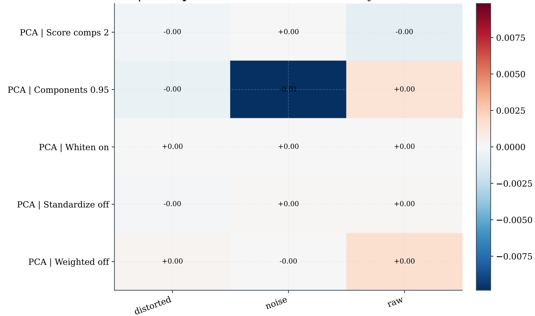
PCA | Mean paired delta in evaluation F1 by dataset variant
