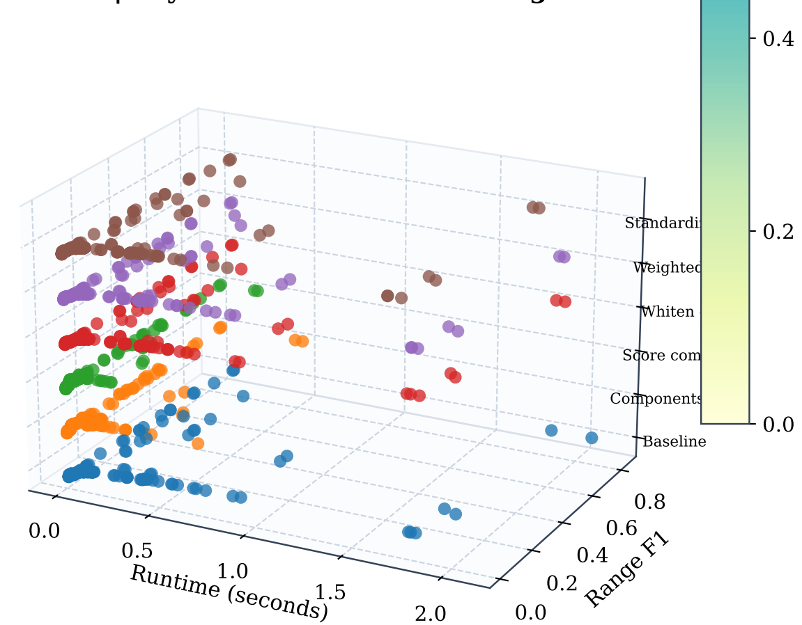
PCA | Layered 3D runtime vs Range F1
