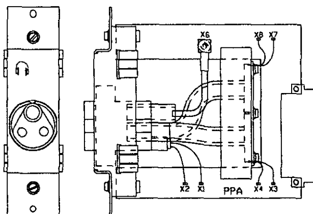
ASSEMBLY HEADINT. (OPTIONAL) (4522 117 8962.)
