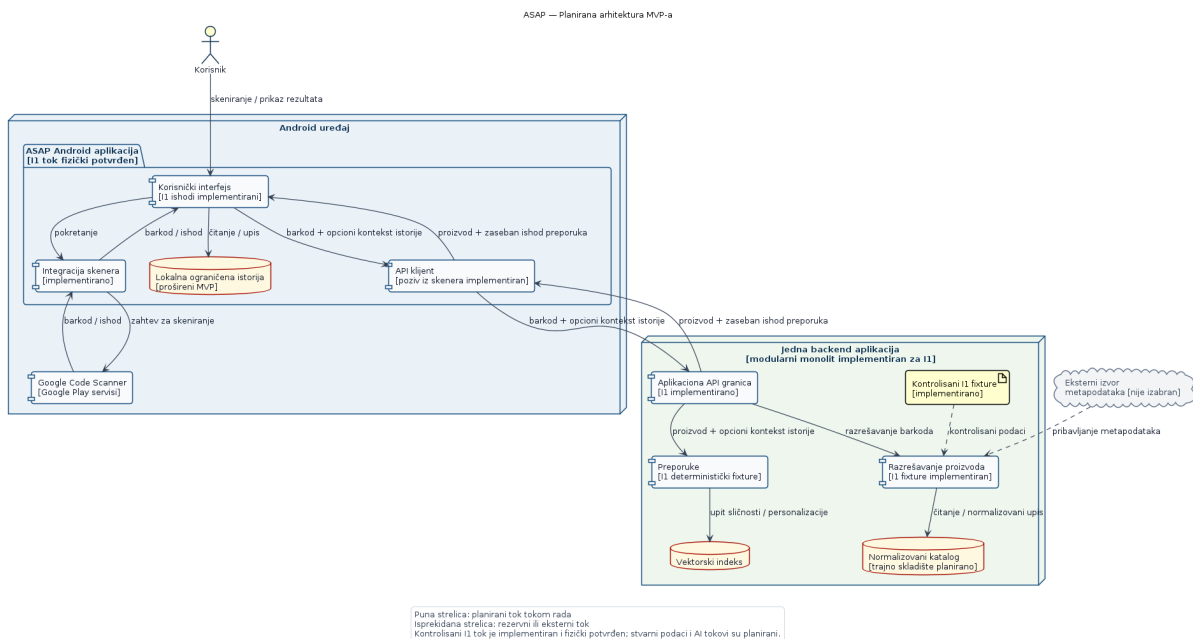
Slika 1: Predložena konkretna arhitektura MVP-a. Kontrolisani I1 tok, od skenera do determinističkog backenda i prikaza ishoda, implementiran je i fizički potvrđen; stvarni podatkovni i AI tokovi predstavljaju plan.
