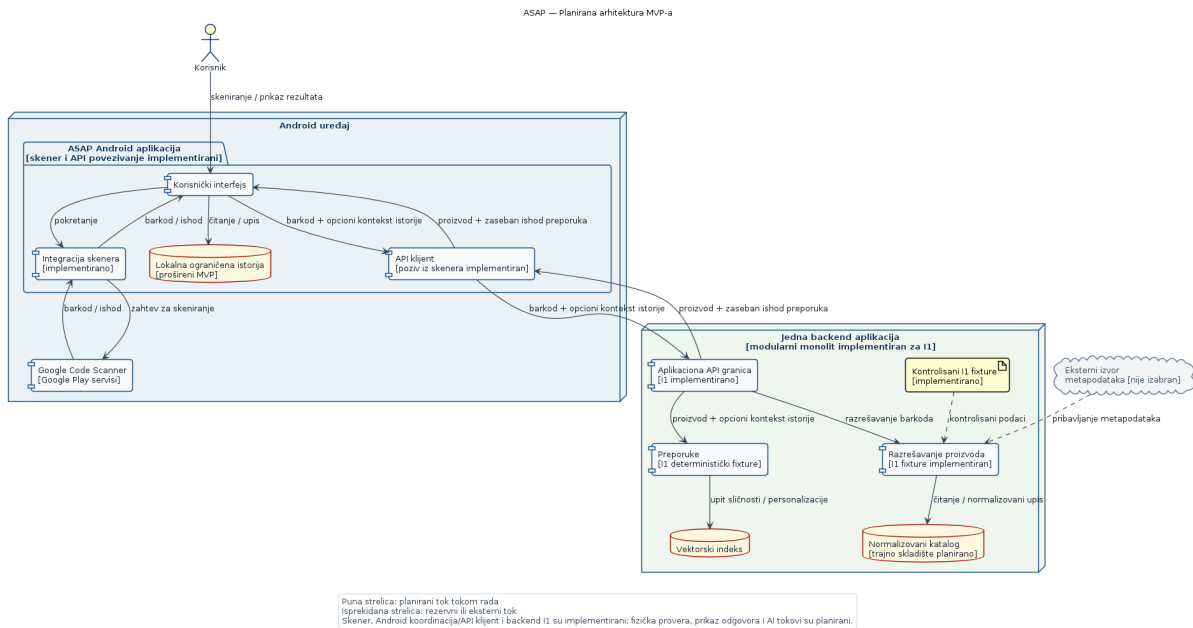
Slika 1: Predložena konkretna arhitektura MVP-a. Skener, Android API povezivanje i deterministički backend I1 su implementirani; fizička provera celog toka, prikaz odgovora i stvarni podatkovni/AI tokovi predstavljaju plan.
