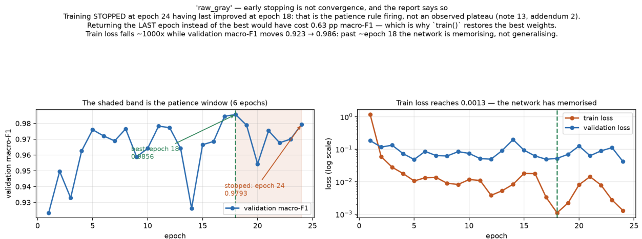
Figure 9: Levo: osenčen pojas je prozor strpljenja. Vraćanje poslednje epohe umesto najbolje koštalo bi 0,63 pp makro-F1. Desno: gubitak nad trening skupom pada oko 1000× dok je validacioni makro-F1 ravan posle epohe 18 – posle te tačke mreža pamti, a ne generalizuje.
