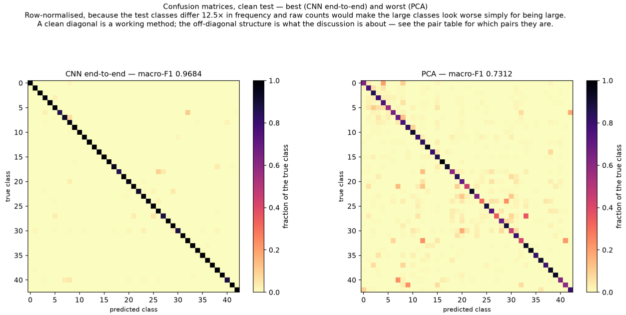
Figure 6: Matrice konfuzije, najbolja i najlošija metoda. Normalizovano po redovima, jer se test klase razlikuju 12,5× po učestanosti, pa bi sirovi brojevi velike klase prikazali lošijim samo zato što su velike.
