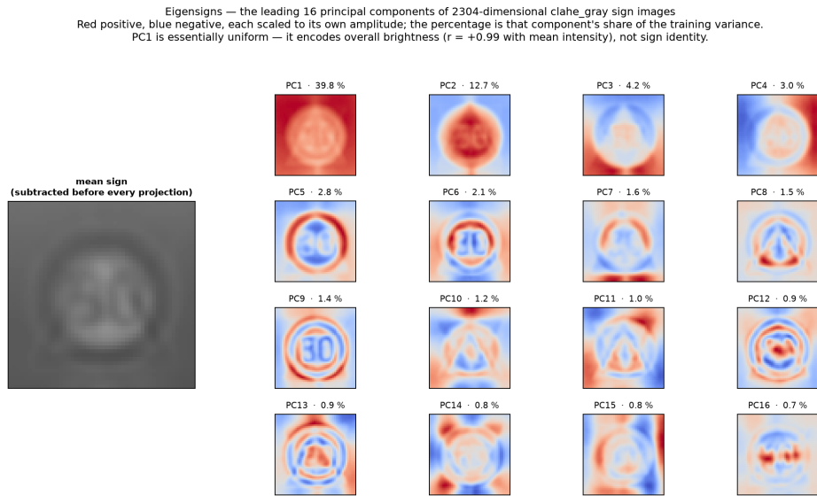
Figure 3: Prvih 16 sopstvenih vektora kao slike („sopstveni znakovi”), sa udelom varijanse. PC1 je osvetljenost (39,8% posle CLAHE), PC2 razlikuje okruglo od trouglastog (12,7%) – najgrublja klasna razlika. Diskriminativni detalj, koja cifra i koji piktogram, živi ispod 1% po komponenti: PCA troši kapacitet po redosledu varijanse, ne po korisnosti.
