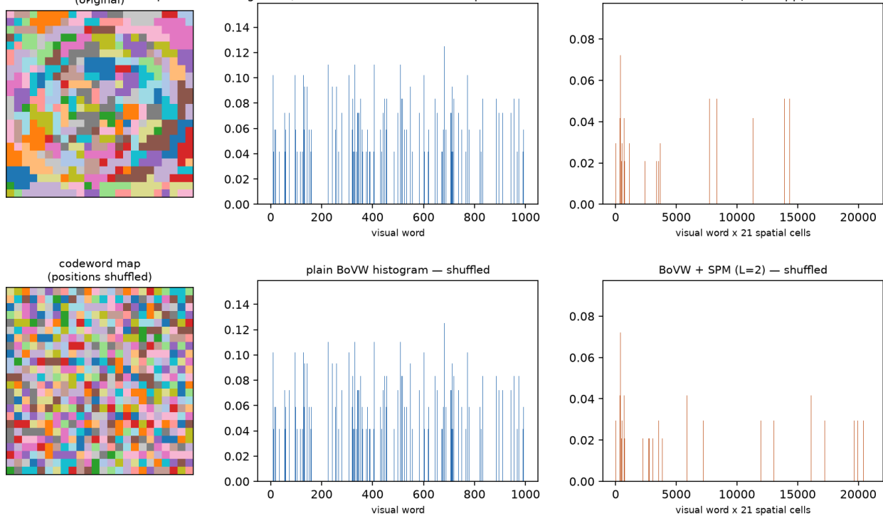
Figure 8: Šta „bez prostornog rasporeda” zaista znači. Isti deskriptori, ponovo sažeti nakon nasumične permutacije njihovih položaja. Obična BoVW: maksimalna razlika 0,0 – to je isti vektor, bit za bitom. Sa piramidom: 0,0833. Karta kodnih reči levo pokazuje da je struktura znaka zaista uništena, a histogram to ne primećuje .
