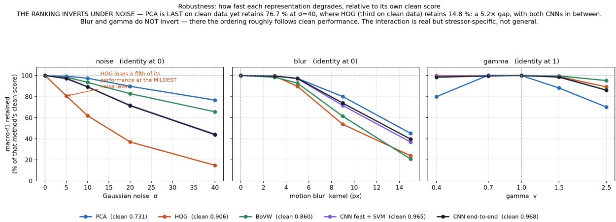
Figure 5: Makro-F1 zadržan u odnosu na sopstvenu čistu vrednost svake metode. Normalizacija je namerna: apsolutne krive su dominirane time odakle svaka metoda kreće, a pitanje ovde nije ko je najbolji – to govori Tabela 1 – već koliko brzo svaka opada .
