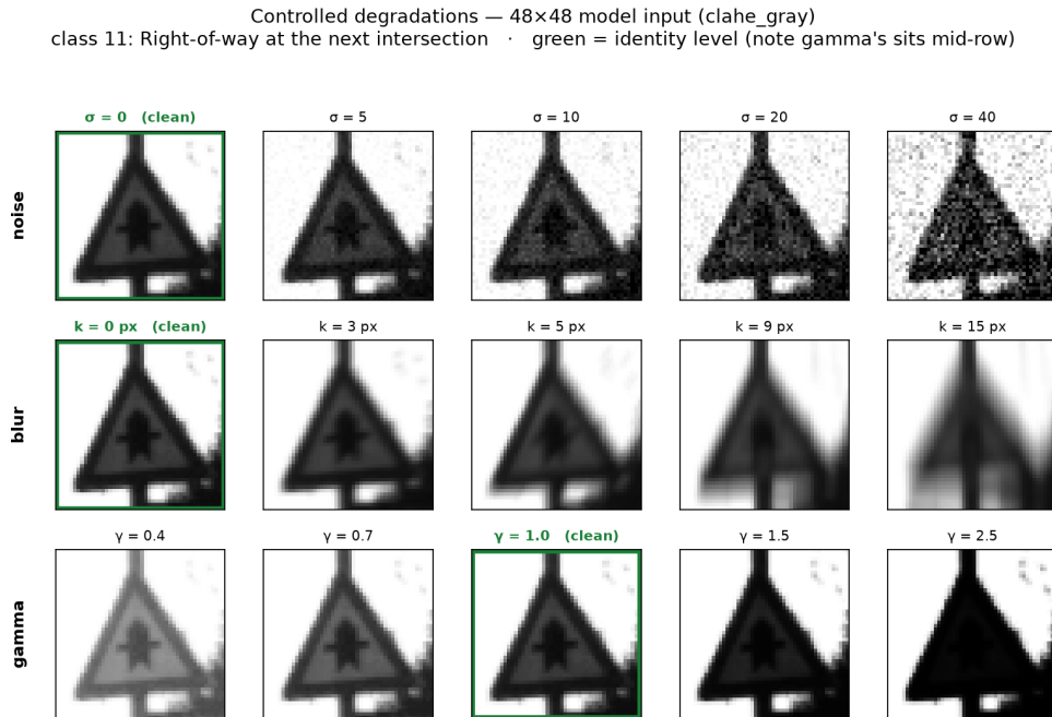
Figure 2: Svaka degradacija na svakom nivou, nad istim uzorkom. Prikazan je stvarni ulaz modela 48 \times 48 ; nivo identiteta je uokviren, a kod gama korekcije se nalazi u sredini reda.
