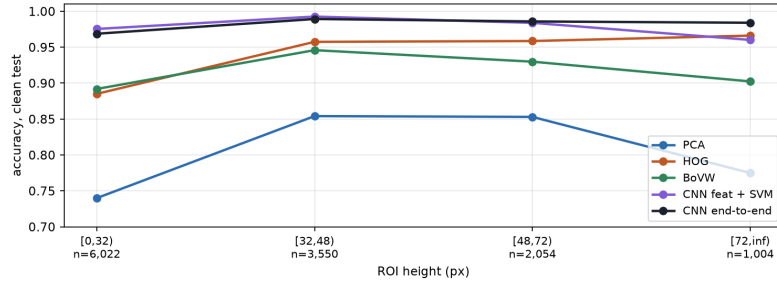
Figure 7: Iste predikcije nad čistim test skupom, grupisane po visini graničnog okvira. Najmanji opseg nije rep raspodele: 47,6% trening slika je ispod 32 px, pa je to modalni slučaj, a raspodele veličina u trening i test skupu se poklapaju na 0,1 pp.
