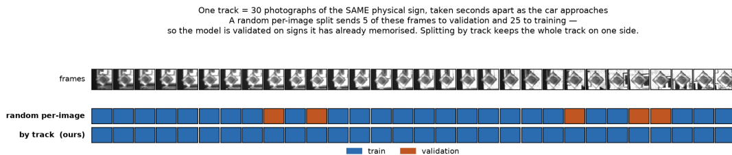
Figure 1: Trideset kadrova jedne sekvence i raspored koji im dodeljuje svako od dva pravila podele. Niz je uređen po rednom broju kadra, pa se čita kao približavanje vozila: kadrovi jesu skoro duplikati, a ne identični, što je razlog zašto ih nijedna provera duplikata ne bi uhvatila. Medijalna korelacija piksela između dva kadra iste sekvence je 0,61 , naspram 0,17 između dve slike iz različitih sekvenci iste klase.
