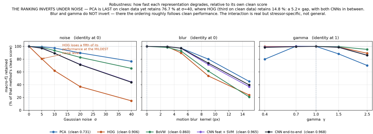
Figure 6: Makro-F1 zadržan u odnosu na sopstvenu čistu vrednost svake metode. Normalizacija je namerna, jer su apsolutne krive dominirane time odakle svaka metoda kreće, a pitanje ovde nije ko je najbolji, o čemu govori Tabela 1, već koliko brzo svaka opada .
