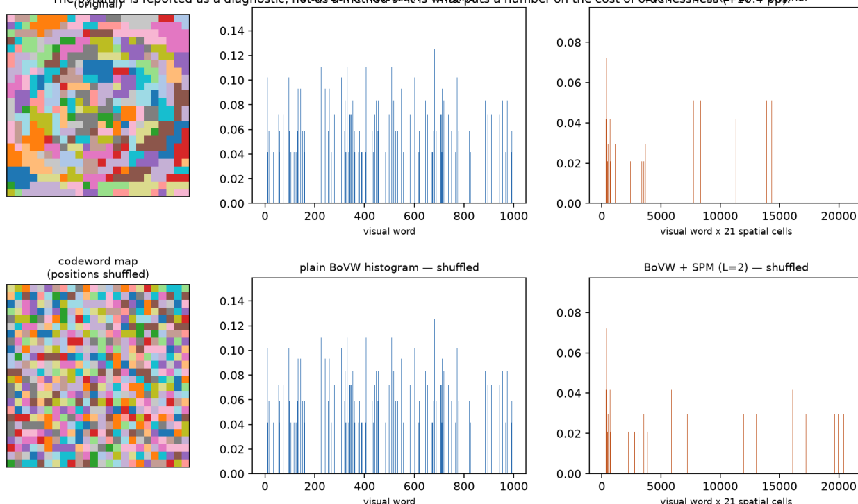
Figure 10: Šta „bez prostornog rasporeda” zaista znači. Isti deskriptori, ponovo sažeti nakon nasumične permutacije njihovih položaja. Kod obične BoVW je maksimalna razlika 0,0, to jest isti vektor, bit-for-bit. Sa piramidom je 0,0833. Karta kodnih reči levo pokazuje da je struktura znaka zaista uništena, a histogram to ne primećuje .
