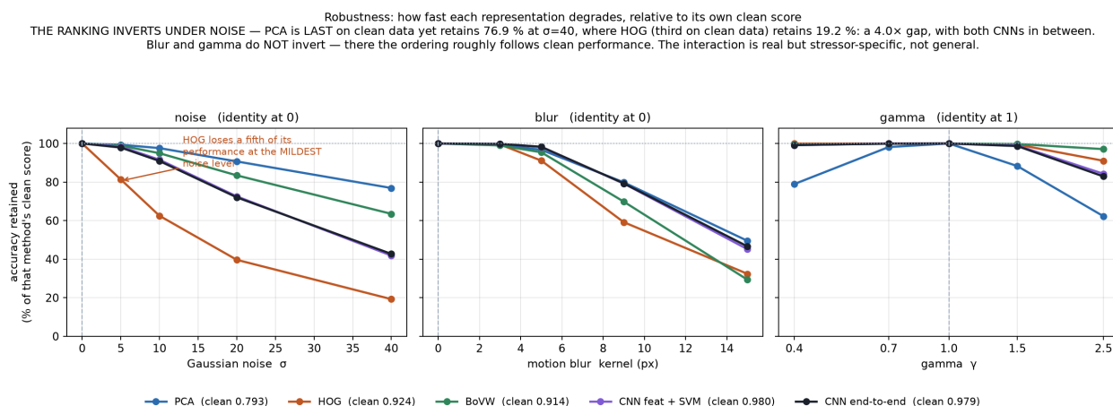
Figure 7: Krive robusnosti po tačnosti, meri koju odeljak 6.3 predloga imenuje. Oblik je isti kao na slici po makro-F1, a razlika je u gama panelu, gde se BoVW i HOG penju iznad obe mreže.
