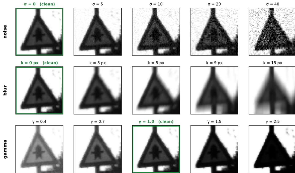
Figure 3: Svaka degradacija na svakom nivou, nad istim uzorkom. Prikazan je stvarni ulaz modela 48 × 48; neutralan nivo je uokviren, a kod gama korekcije se nalazi u sredini reda.
