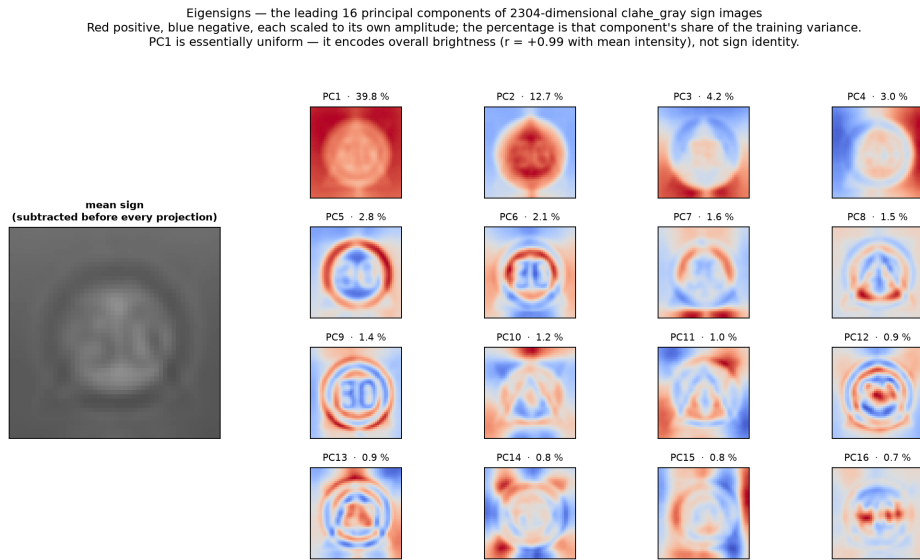
Figure 4: Prvih 16 sopstvenih vektora kao slike („sopstveni znakovi”), sa udelom varijanse. PC1 je osvetljenost (39,8% posle CLAHE), PC2 razlikuje okruglo od trouglastog (12,7%), što je najgrublja klasna razlika. Diskriminativni detalj, koja cifra i koji piktogram, živi ispod 1% po komponenti. PCA troši kapacitet po redosledu varijanse, ne po korisnosti.
