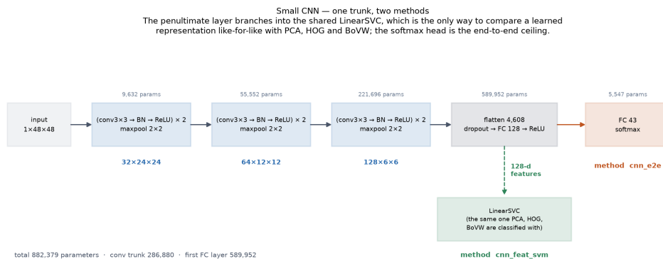
Figure 5: Dva izlaza jedne mreže — softmax glava daje cnn_e2e , a preposlednji sloj se grana u zajednički linearni SVM i daje cnn_feat_svm . U celom projektu postoji tačno jedno treniranje mreže, jer cnn_feat_svm ne trenira ništa novo.
