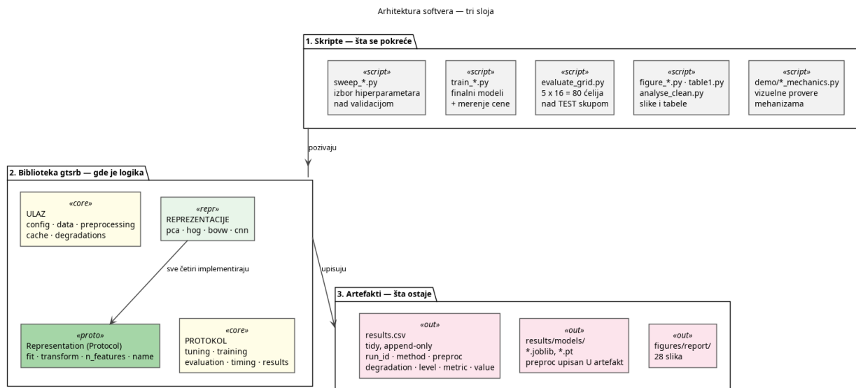
Figure 1: Tri sloja — skripte pozivaju biblioteku, biblioteka upisuje artefakte. Strelice su agregirane radi čitljivosti, jer svaka skripta koristi više modula.
