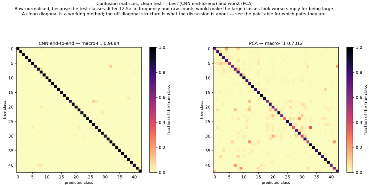
Slika 8: Matrice konfuzije, najbolja i najlošija metoda. Normalizovano po redovima, jer se test klase razlikuju 12,5x po učestanosti, pa bi sirovi brojevi velike klase prikazali lošijim samo zato što su velike.
