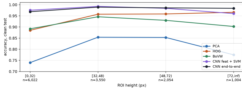
Slika 9: Iste predikcije nad čistim test skupom, grupisane po visini graničnog okvira. Najmanji opseg nije rep raspodele, jer je 47,6% trening slika je ispod 32 px, pa je to modalni slučaj, a raspodele veličina u trening i test skupu se poklapaju na 0,1 pp.
