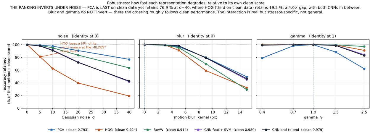
Slika 7: Krive robusnosti po tačnosti, meri koju odeljak 6.3 predloga imenuje. Oblik je isti kao na slici po makro-F1, a razlika je u gama panelu, gde se BoVW i HOG penju iznad obe mreže.
