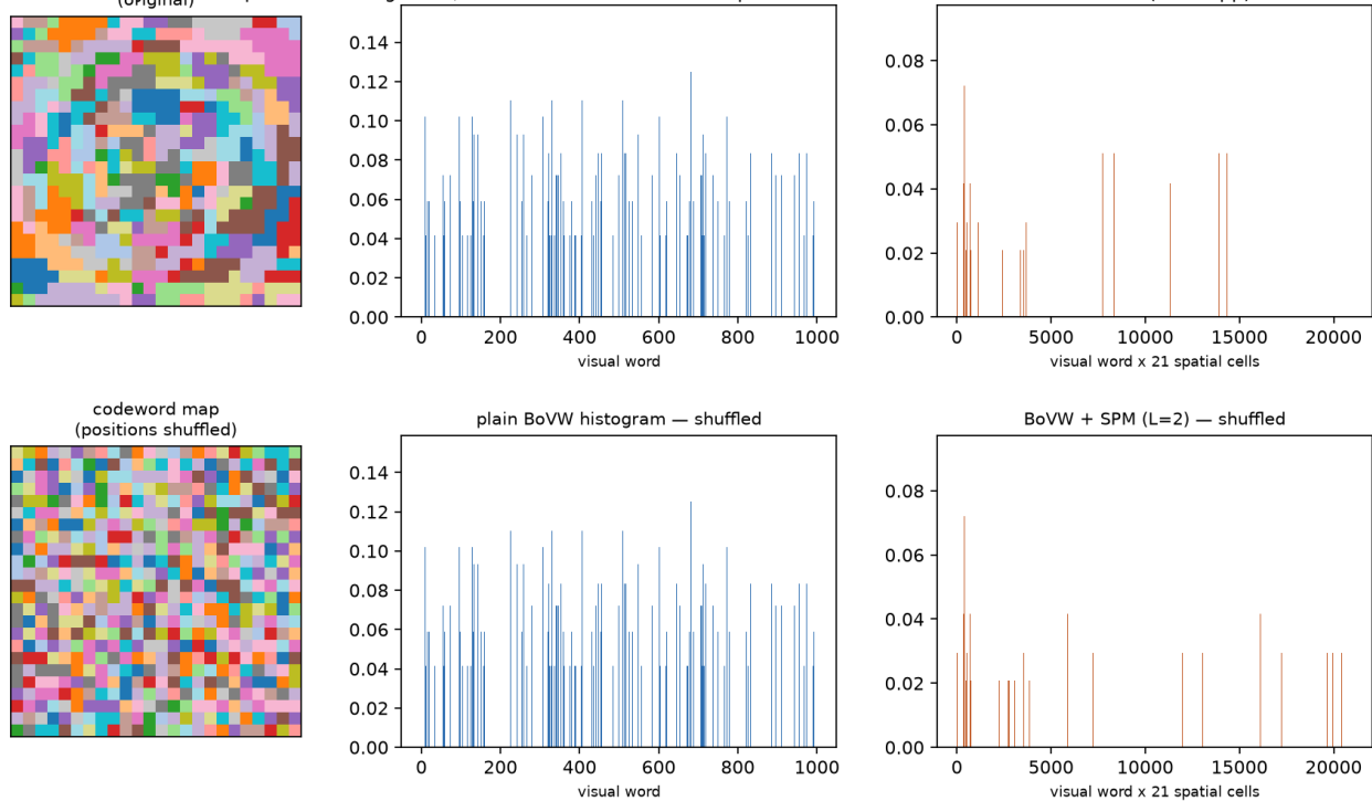
Figure 9: Šta „bez prostornog rasporeda” zaista znači. Isti deskriptori, ponovo sažeti nakon nasumične permutacije njihovih položaja. Obična BoVW: maksimalna razlika 0,0 – to je isti vektor, bit-for-bit . Sa piramidom: 0,0833. Karta kodnih reči levo pokazuje da je struktura znaka zaista uništena, a histogram to ne primećuje .
