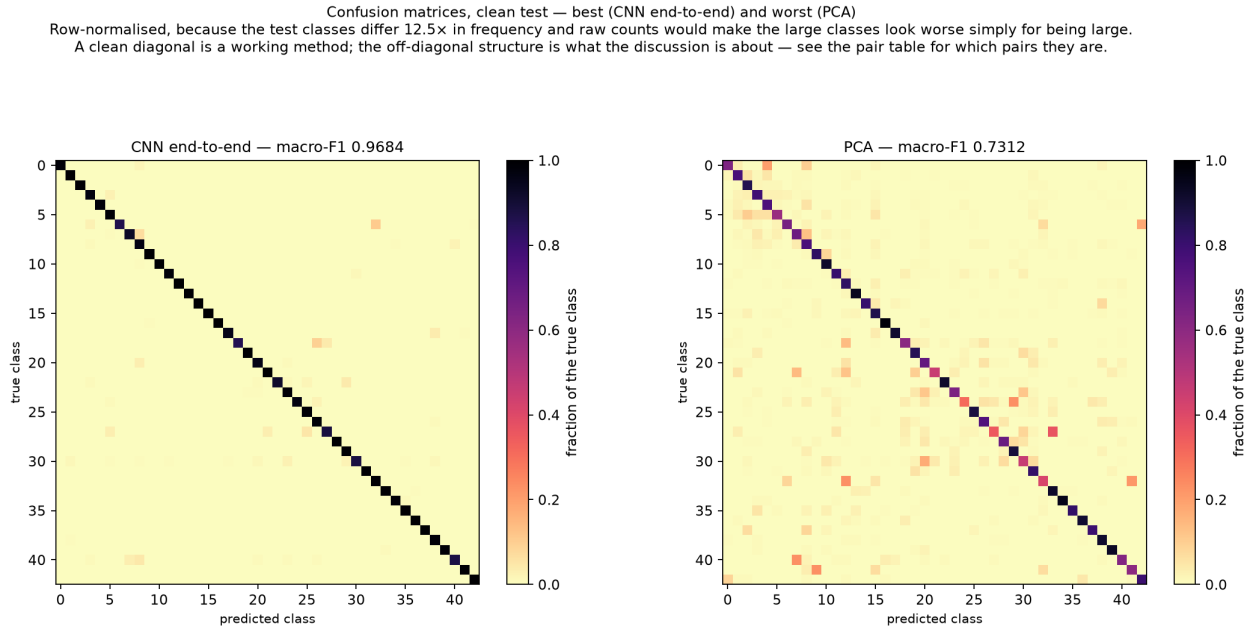
Figure 7: Matrice konfuzije, najbolja i najlošija metoda. Normalizovano po redovima, jer se test klase razlikuju 12,5x po učestanosti, pa bi sirovi brojevi velike klase prikazali lošijim samo zato što su velike.
