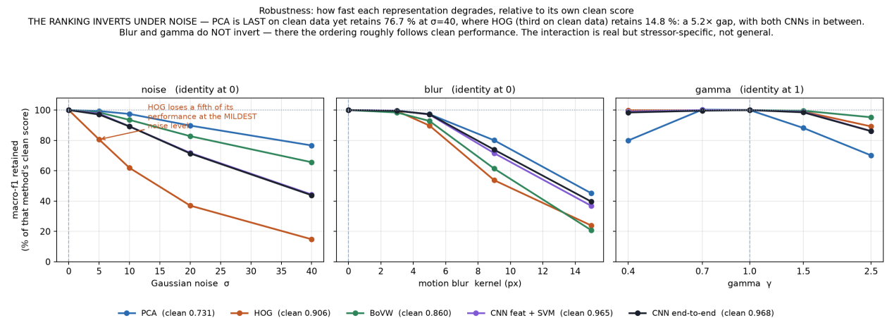
Figure 5: Makro-F1 zadržan u odnosu na sopstvenu čistu vrednost svake metode. Normalizacija je namerna: apsolutne krive su dominirane time odakle svaka metoda kreće, a pitanje ovde nije ko je najbolji – to govori Tabela 1 – već koliko brzo svaka opada .
