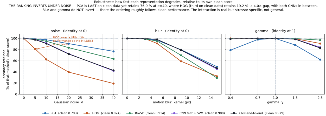
Figure 6: Krive robusnosti po tačnosti – mera koju odeljak 6.3 predloga imenuje. Oblik je isti kao na slici po makro-F1, a razlika je u gama panelu, gde se BoVW i HOG penju iznad obe mreže.
