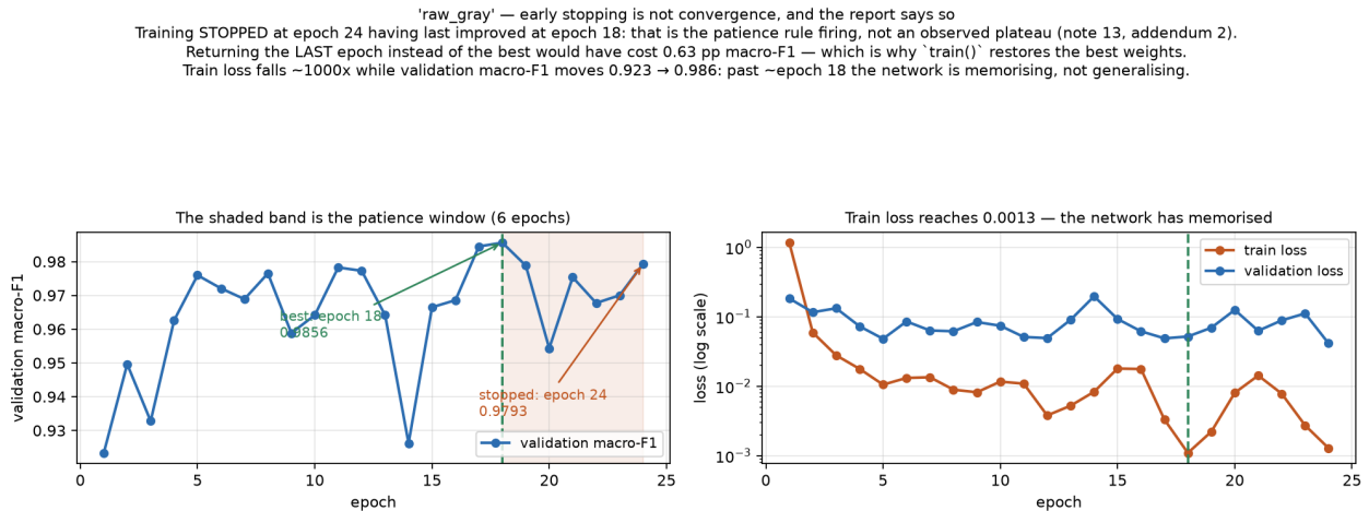
Figure 10: Levo: osenčen pojas je patience prozor. Vraćanje poslednje epohe umesto najbolje koštalo bi 0,63 pp makro-F1. Desno: gubitak nad trening skupom pada oko 1000× dok je validacioni makro-F1 ravan posle epohe 18 – posle te tačke mreža pamti, a ne generalizuje.
