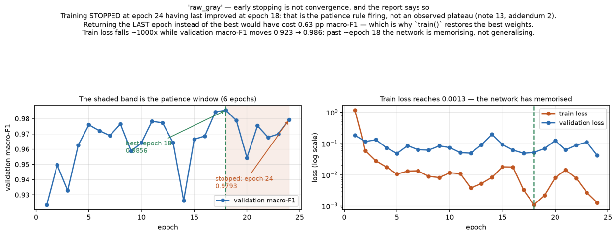
Figure 9: Levo: osenčen pojas je patience prozor. Vraćanje poslednje epohe umesto najbolje koštalo bi 0,63 pp makro-F1. Desno: gubitak nad trening skupom pada oko 1000\times dok je validacioni makro-F1 ravan posle epohe 18 – posle te tačke mreža pamti, a ne generalizuje.
