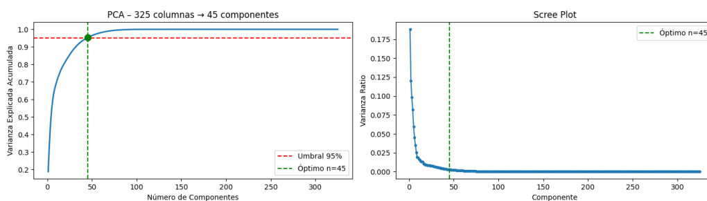
Figura 3.11: Reducción de características
