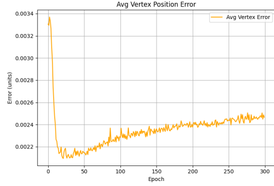
Figura 3.9: Visualización del error medio a lo largo del entrenamiento
