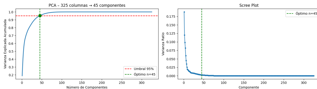
Figura 3.12: Ejemplo de componentes óptimos para PCA
