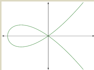
Figura 3: Gráfica de la curva elíptica Curve25519 .
