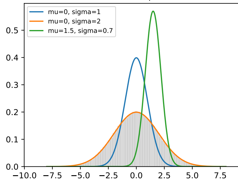
Gaussian pdf
