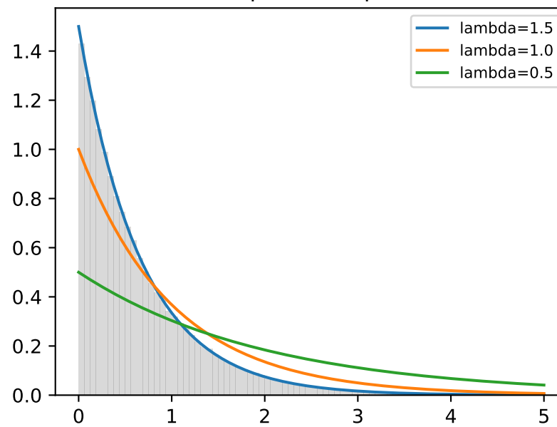
Exponential pdf
