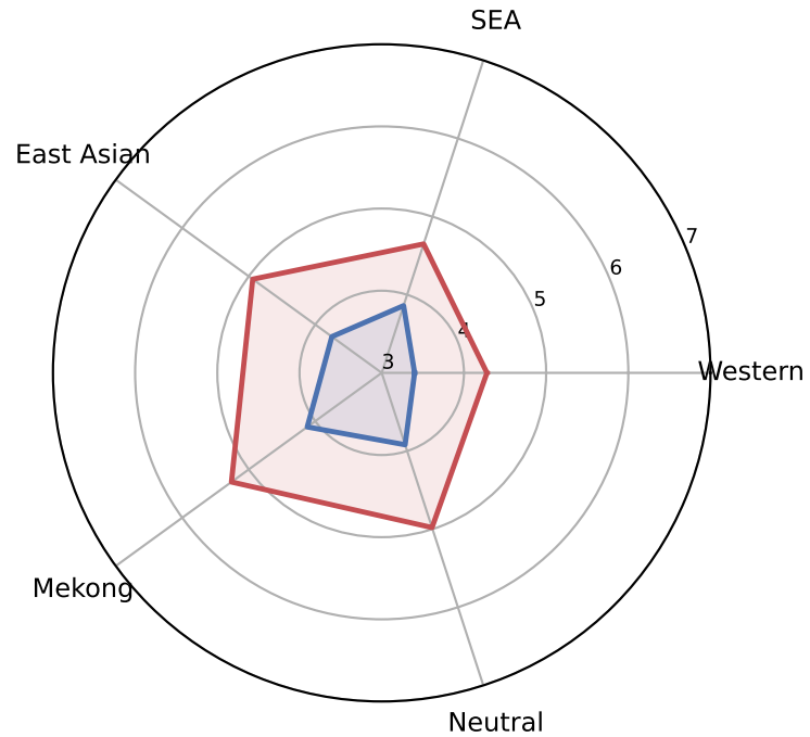
Claude Sonnet
