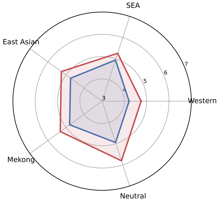
GPT-4o
