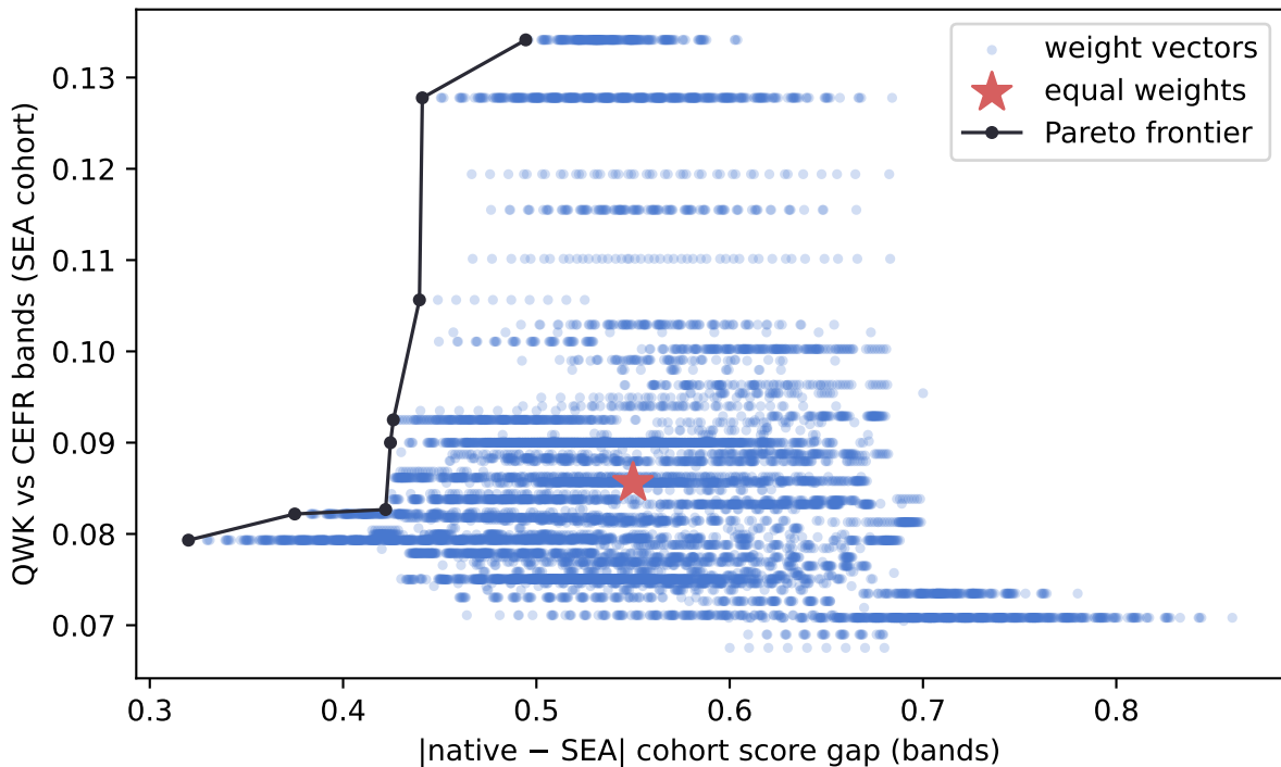
Fairness-accuracy frontier: gpt-4o
