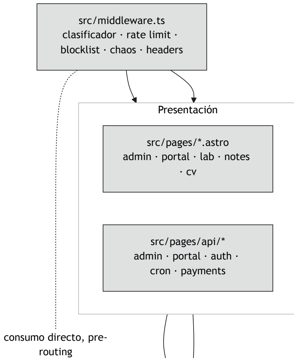
Figura 21 (sección 1 de 3) Diagrama de paquetes
