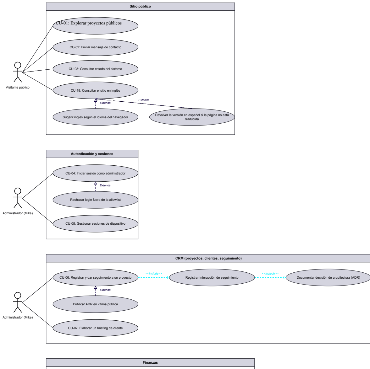
Figura 1 (sección 1 de 3) Diagrama de casos de uso
