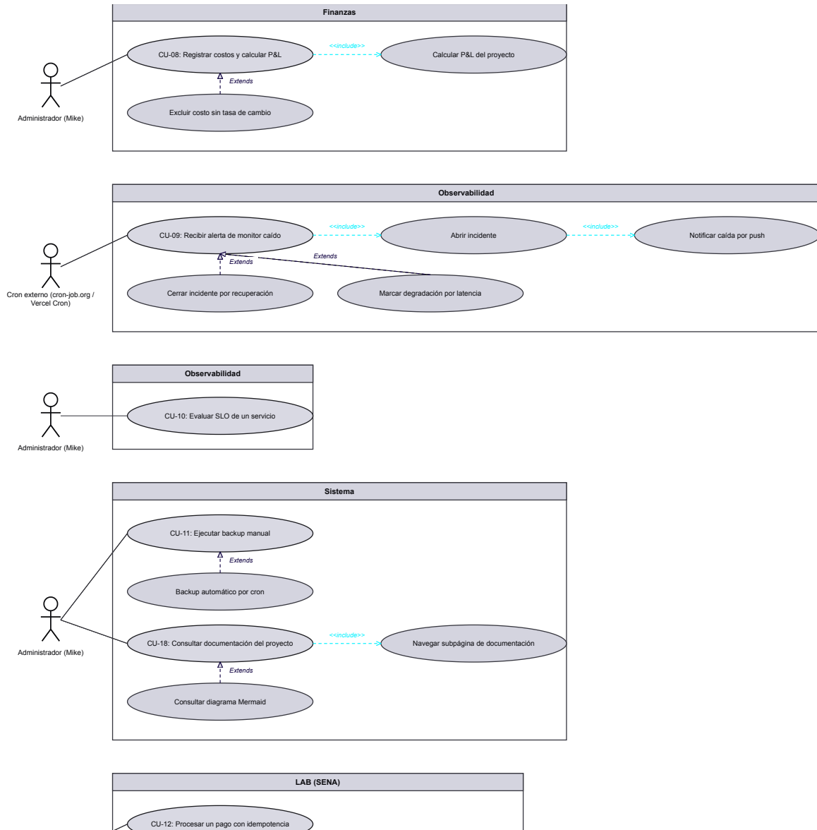
Figura 1 (sección 2 de 3) Diagrama de casos de uso
