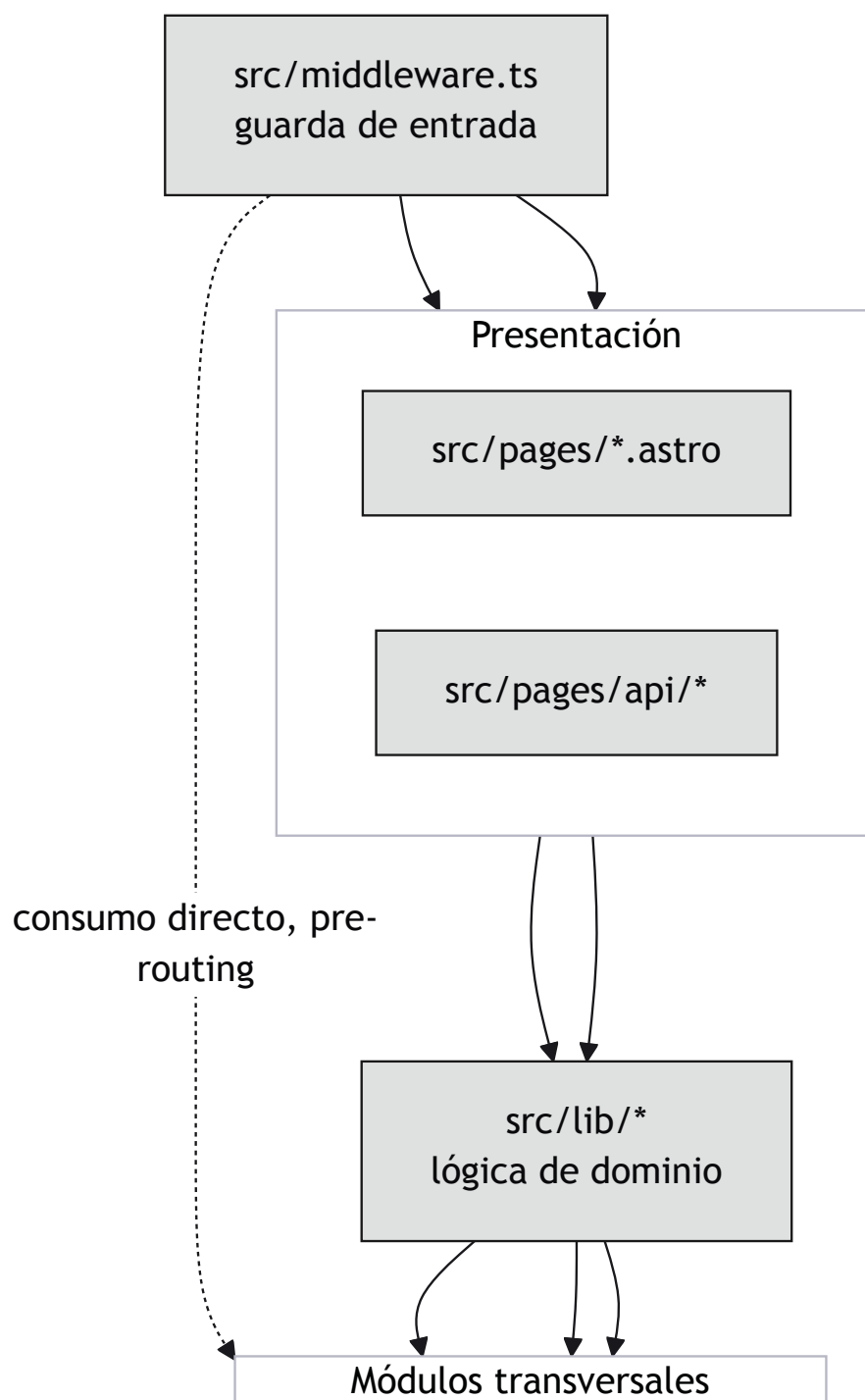
Figura 28 (sección 1 de 2) Diagrama de paquetes
