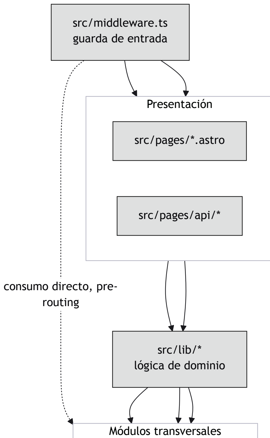
Figura 31 (sección 1 de 2) Diagrama de paquetes
