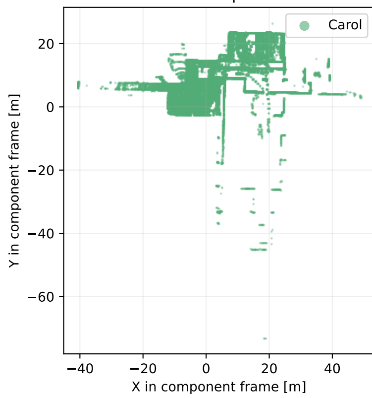
Raw BEVs · component Carol
