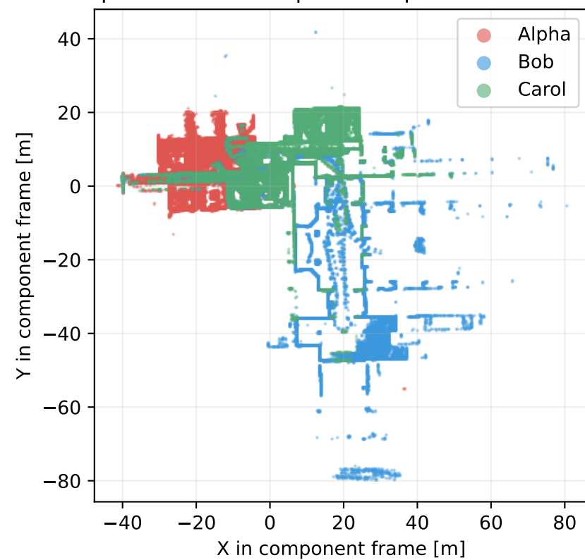
Ellipsoid BEVs · component Alpha + Bob + Carol
