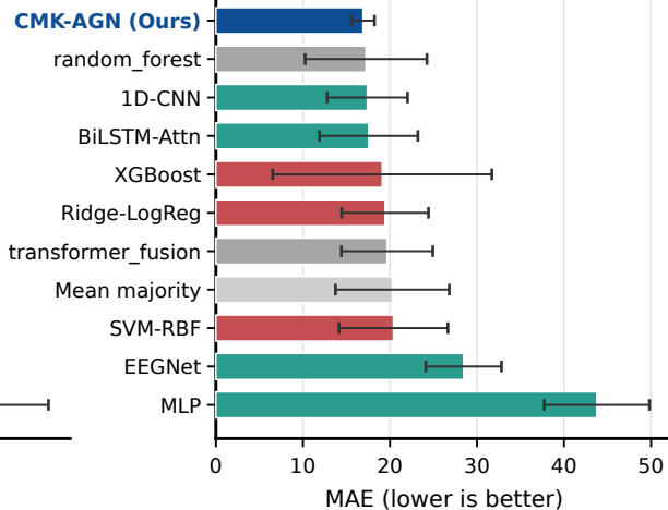
(b) BI
