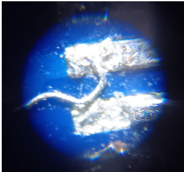
Abbildung 4: Lötbrücke bei einem der LQFP48-Pins des STM32G431
