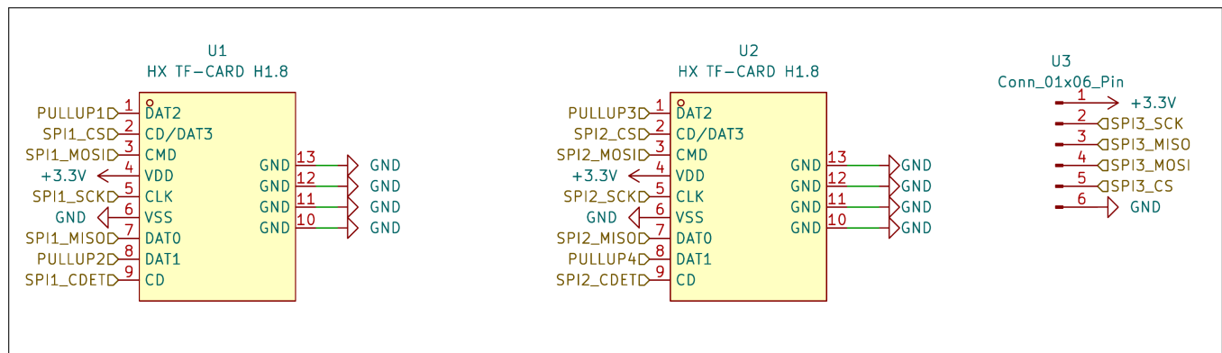
Abbildung 2: Schaltplan für die SPI-Interfaces
