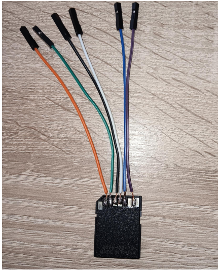
Abbildung 7: Erster gelöteter SD-Adapter
