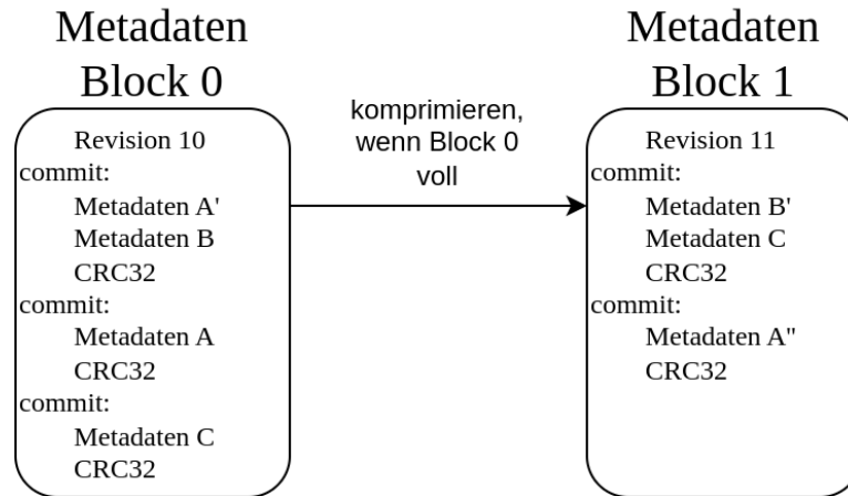
Abbildung 17: Prinzip „two-block log“
