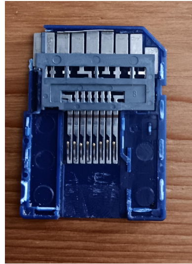
Abbildung 8: Aufgebrochener SD-Adapter
