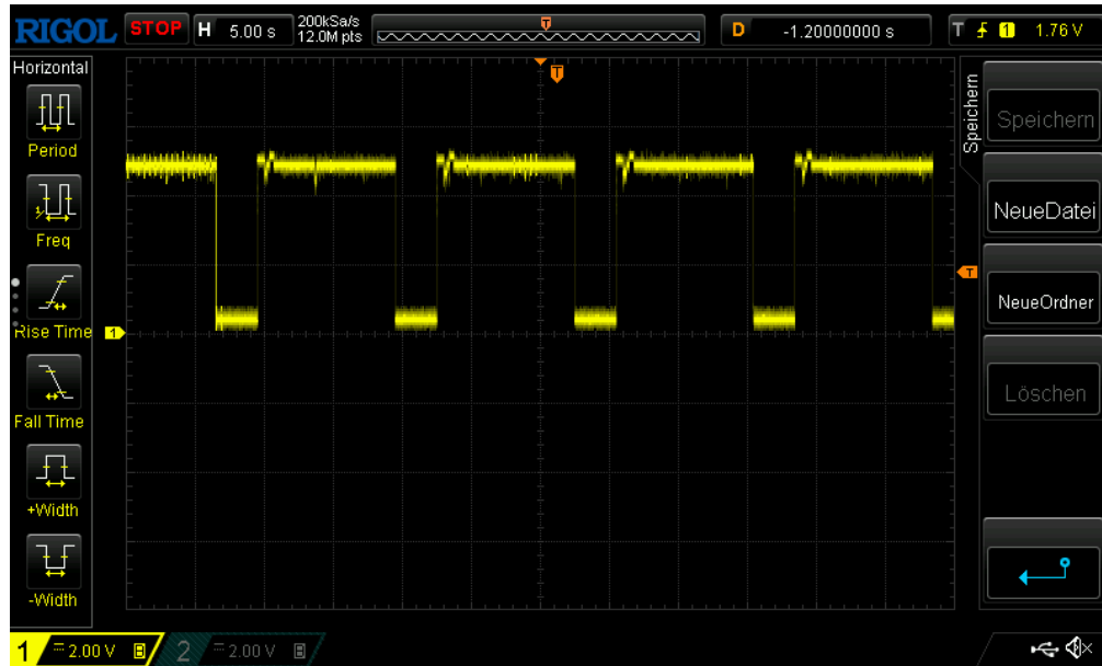
Abbildung 22: Verifizierung der Spannung am LDO-Eingang
