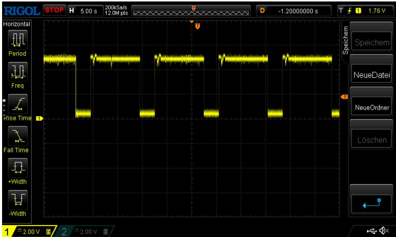
Abbildung 25: Verifizierung der Spannung am LDO-Eingang
