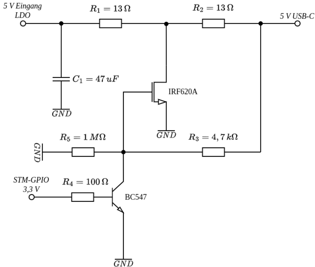
Abbildung 23: „killswitch“-Schaltung für eine periodische Unterbrechung der Spannungsversorgung
