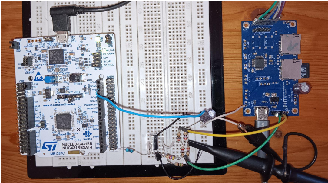
Abbildung 24: Aufbau der „killswitch“-Schaltung auf einem Steckbrett
