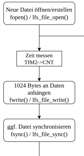
Abbildung 26: Schleife für das Anhängen von 1024 Byte an eine Versuchsdatei
