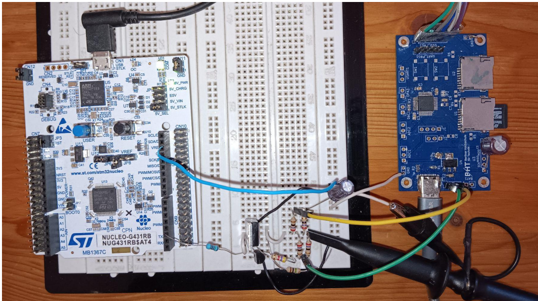
Abbildung 30: Aufbau der „killswitch“-Schaltung auf einem Steckbrett
