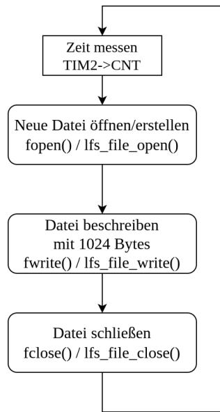
Abbildung 21: Schreibzyklus für eine 1024 Byte große Versuchsdatei
