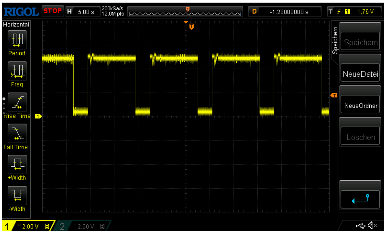
Abbildung 31: Verifizierung der Spannung am LDO-Eingang
