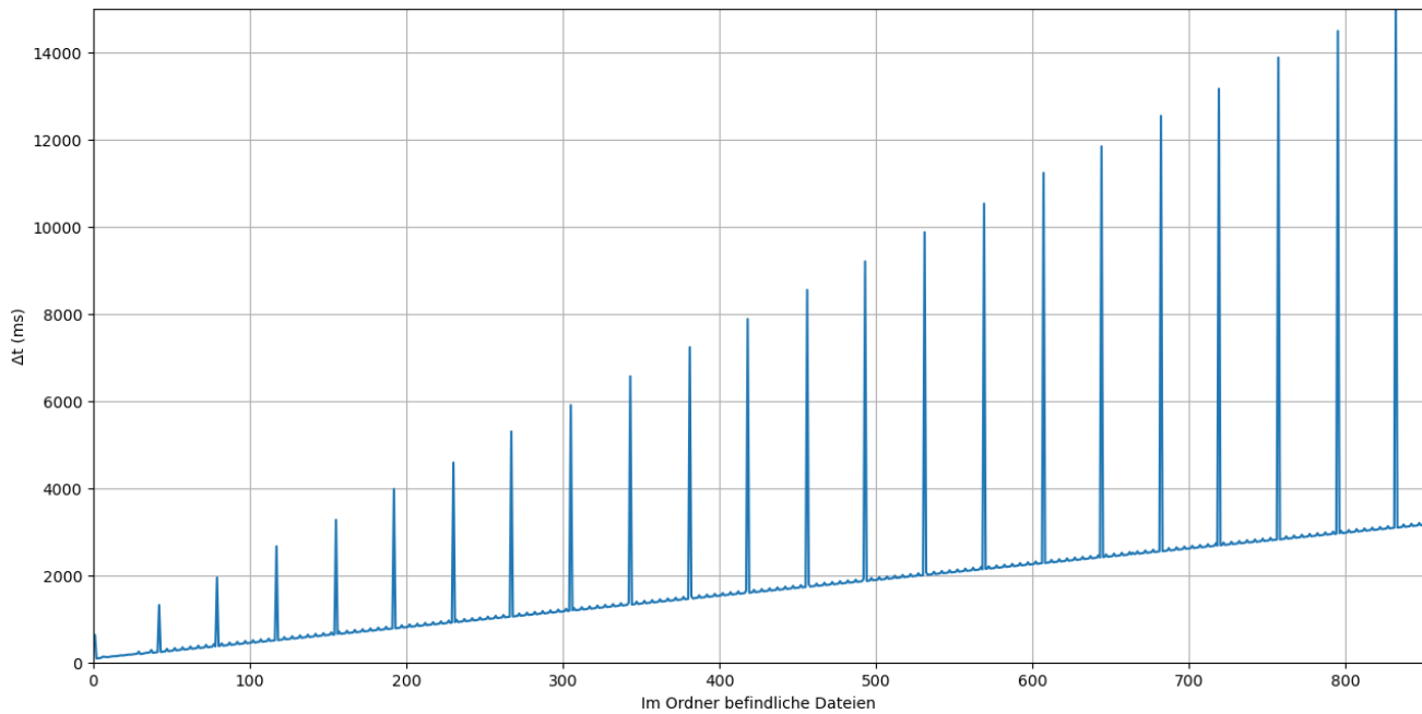
Abbildung 23: Dauer der Neuerstellung von 1 KB Dateien auf dem littlefs-Dateisystem
