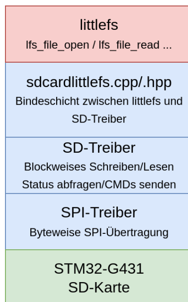
Abbildung 20: Implementierungsstack für das littlefs-Dateisystem
