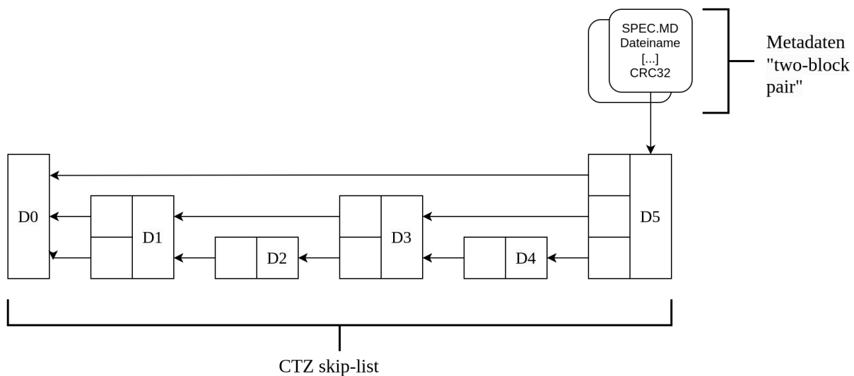
Abbildung 19: Prinzip des Dateiaufbaus bei littlefs
