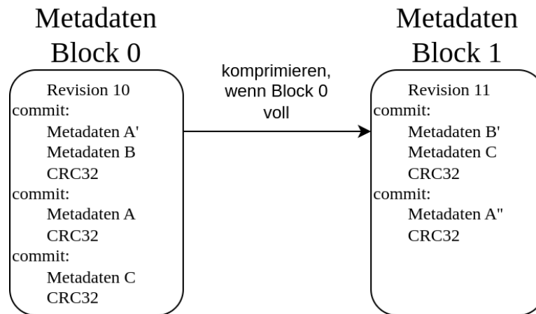
Abbildung 18: Prinzip „two-block log“
