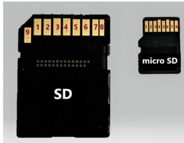
Abbildung 9: Pinnummerierung SD-Karten[15]
