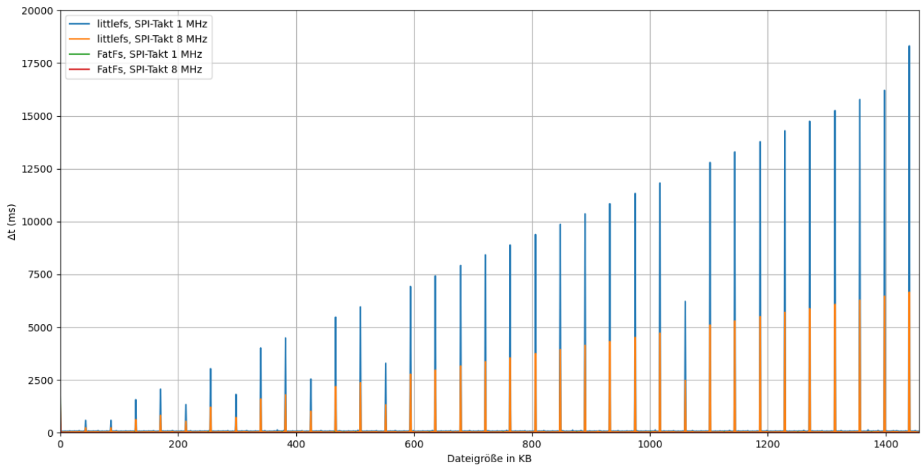
Abbildung 28: Dauer des Anhängens von 1 KB an eine Datei in Abhängigkeit der Dateigröße
