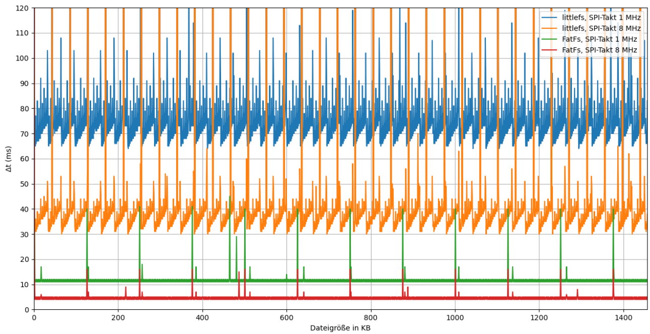
Abbildung 27: Dauer des Anhängens von 1 KB an eine Datei in Abhängigkeit der Dateigröße
