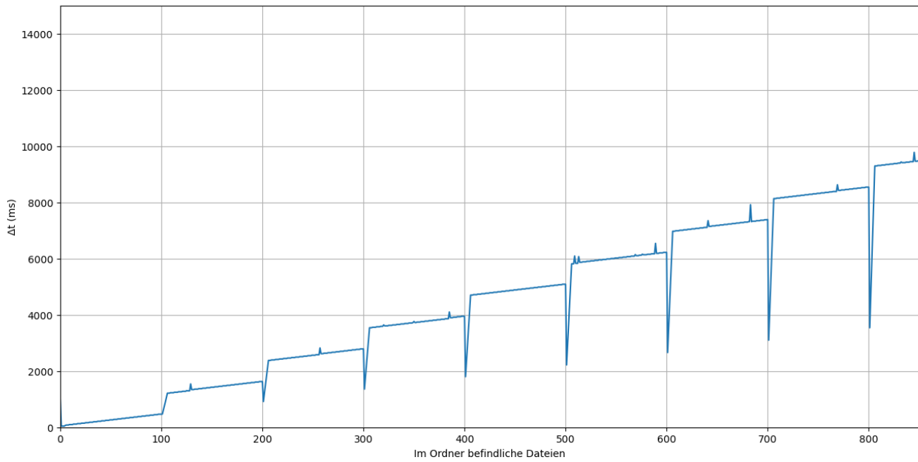
Abbildung 22: Dauer der Neuerstellung von 1 KB Dateien auf dem FatFs-Dateisystem
