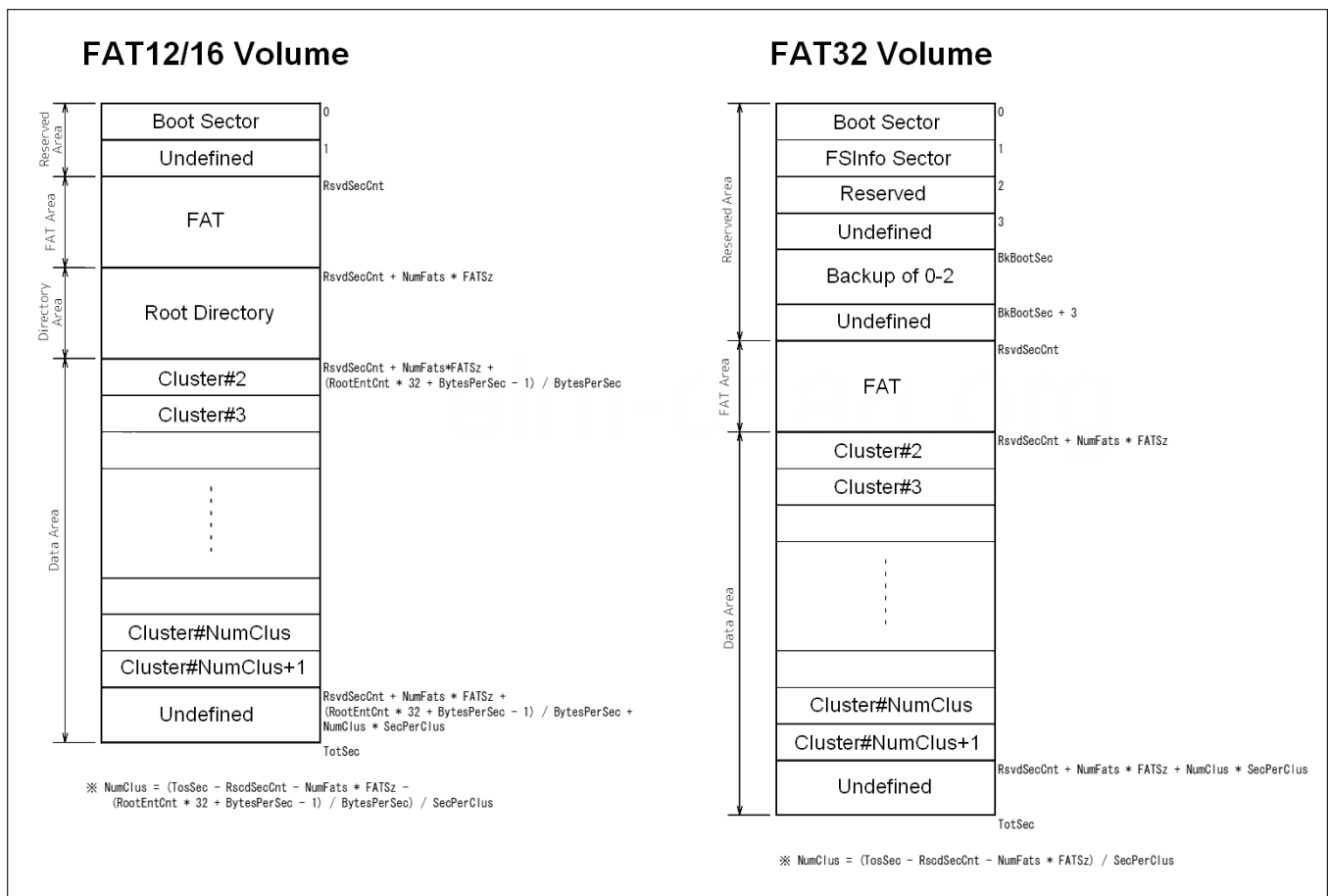
Abbildung 16: Struktur der FAT-Dateisysteme [9]
