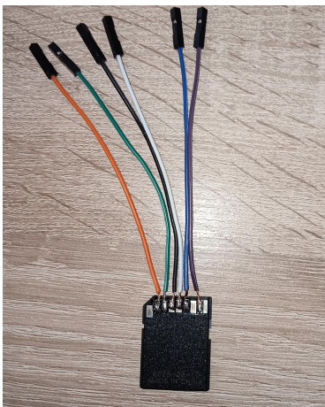
Abbildung 7: Erster gelöteter SD-Adapter
