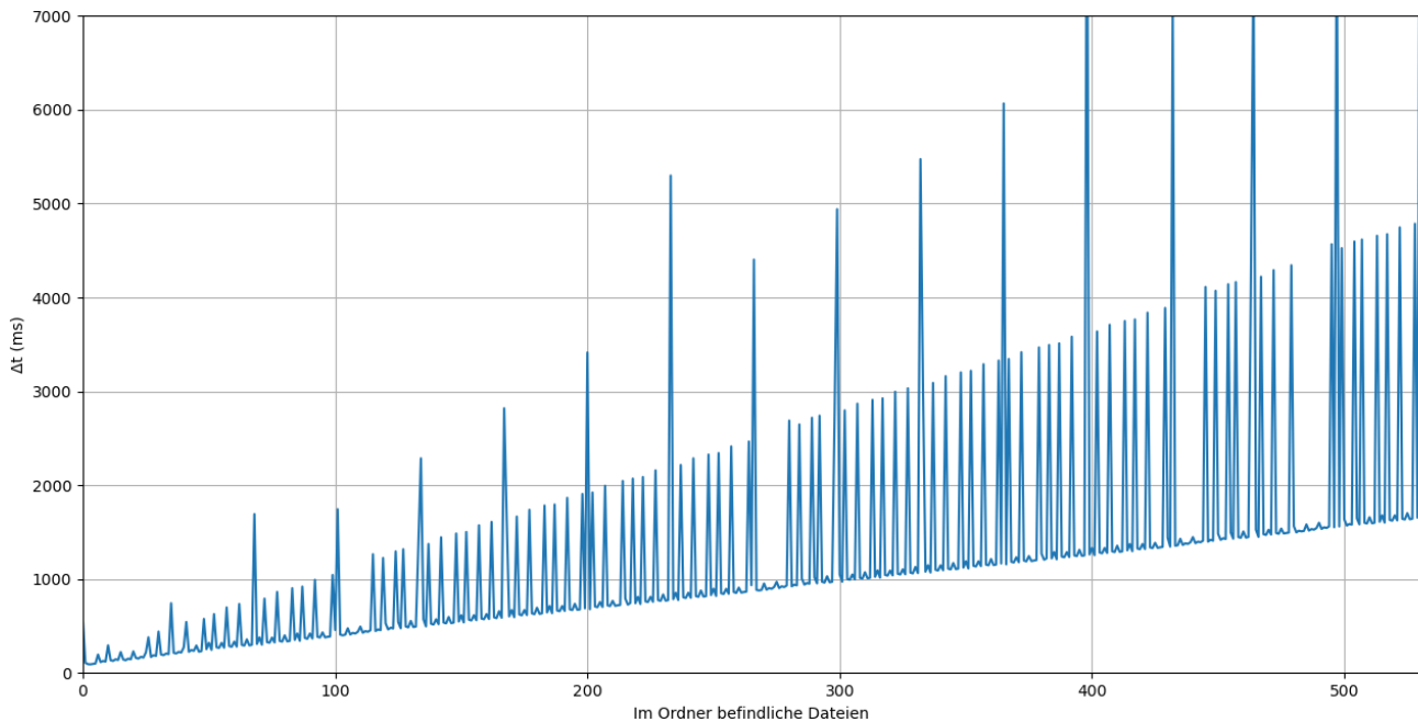
Abbildung 24: Dauer der Neuerstellung von Dateien auf dem littlefs-Dateisystem mit korrupten Daten
