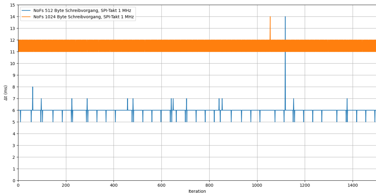
Abbildung 32: Dauer von 512 Byte und 1024 Byte Schreibvorgängen
