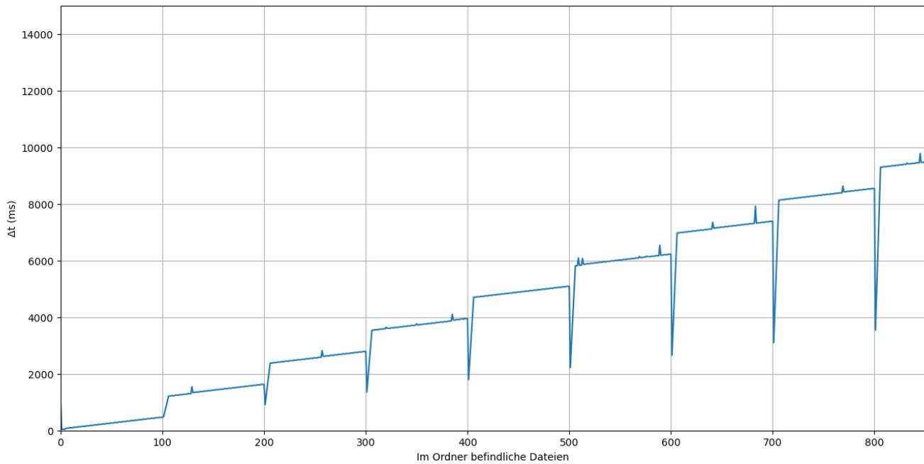
Abbildung 22: Dauer der Neuerstellung von Dateien auf dem FatFs-Dateisystem
