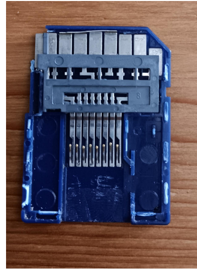
Abbildung 8: Aufgebrochener SD-Adapter
