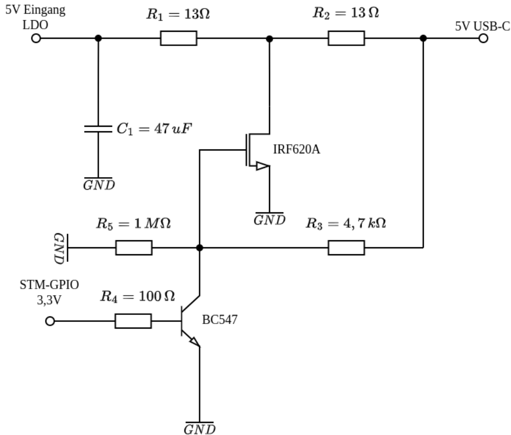
Abbildung 20: „killswitch“-Schaltung für eine periodische Unterbrechung der Spannungsversorgung
