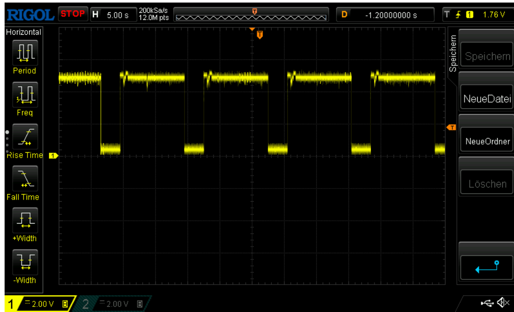
Abbildung 22: Verifizierung der Spannung am LDO-Eingang
