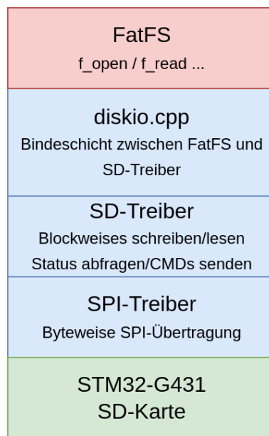
Abbildung 13: Implementierungsstack für das FatFS-Dateisystem
