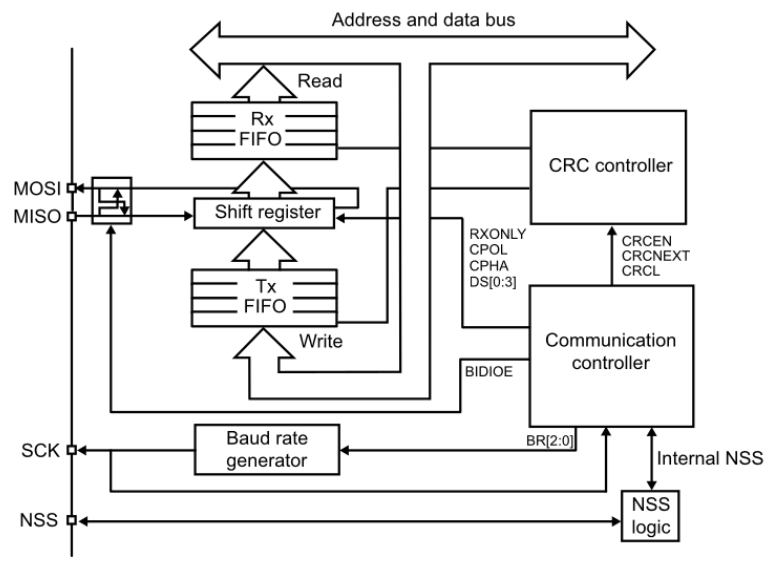
Abbildung 10: Blockdiagramm für die SPI-Peripherie des STMG431[4]
