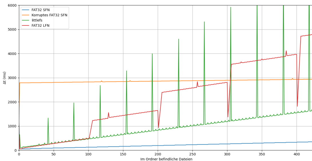
Abbildung 22: Dauer der Neuerstellung von Dateien Übersicht
