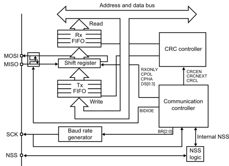
Abbildung 10: Blockdiagramm für die SPI-Peripherie des STM32G431[?]
