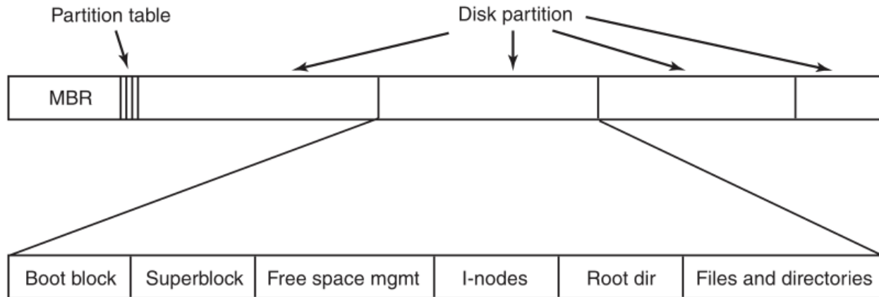
Abbildung 12: Ein mögliches Dateisystemlayout [?, S. 282]
