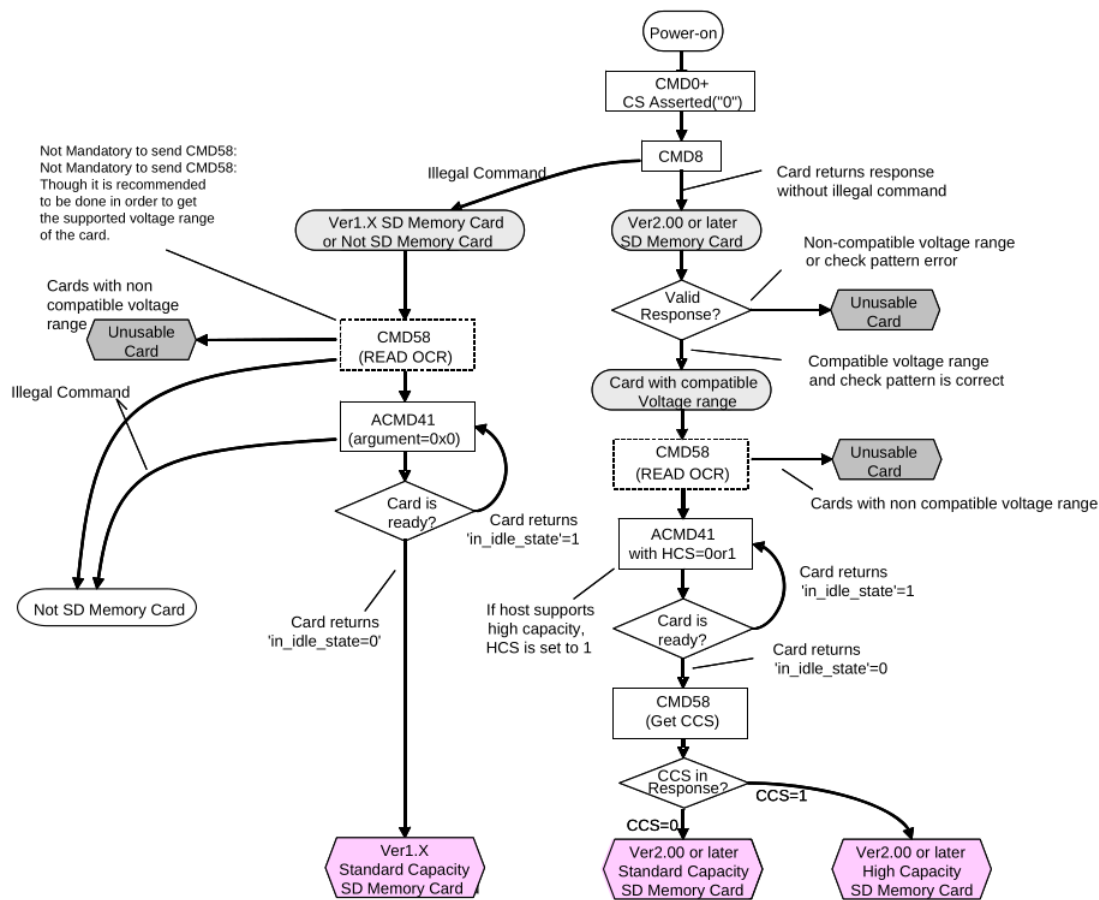
Abbildung 11: Initialisierung der SD-Karte in den SPI-Modus[?]
