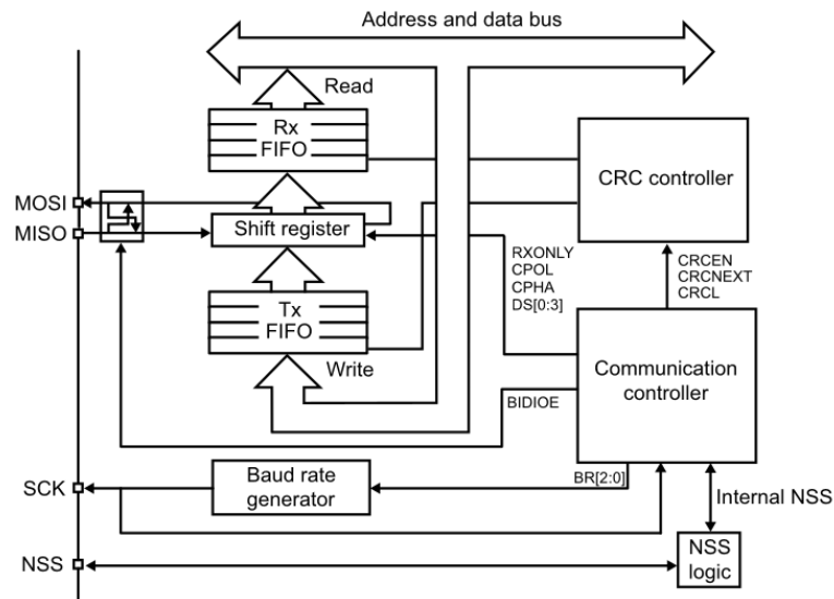
Abbildung 11: Blockdiagramm für die SPI-Peripherie des STM32G431[4]
