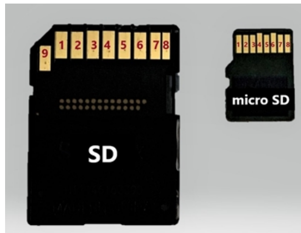
Abbildung 10: Pinnummerierung SD-Karten[13]
