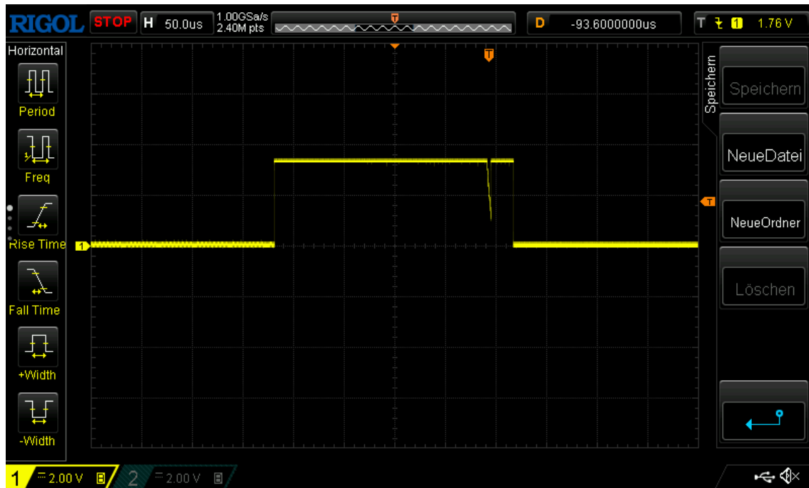
Abbildung 7: MISO: SD-Kartenantwort auf CMD0
