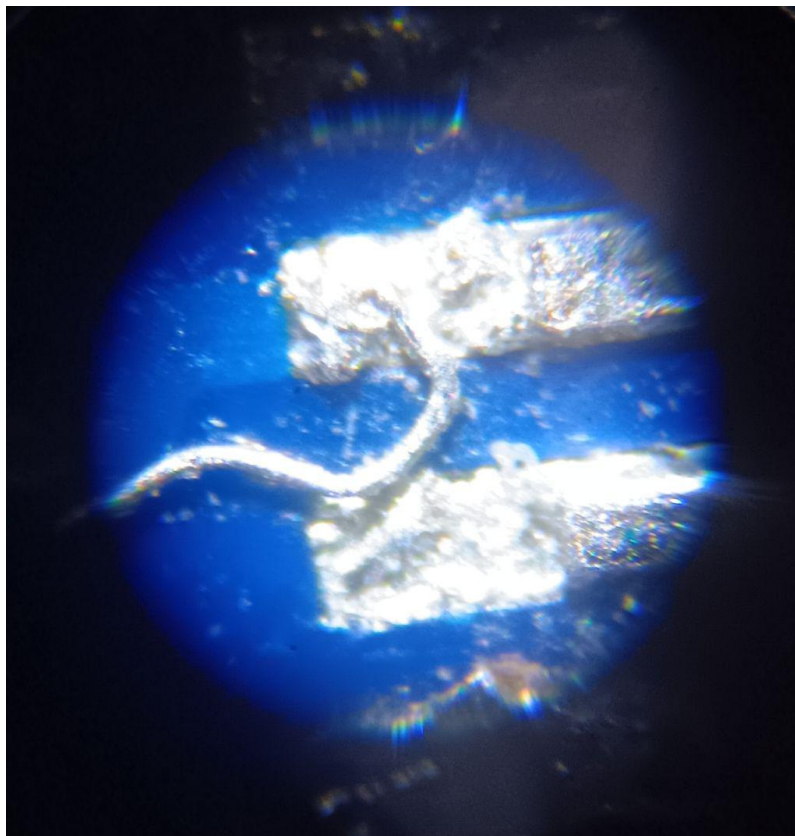
Abbildung 5: Lötbrücke bei einem der LQFP48-Pins des STM32G431
