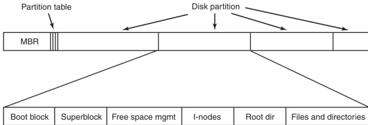
Abbildung 5: Ein mögliches Dateisystemlayout [1, S. 282]
