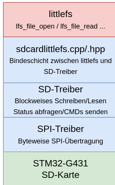
Abbildung 17: Implementierungsstack für das littlefs-Dateisystem
