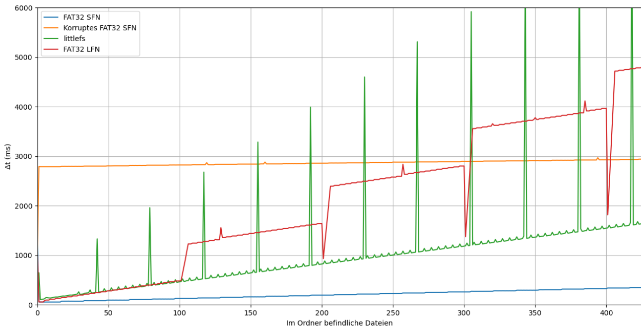
Abbildung 22: Dauer der Neuerstellung von Dateien Übersicht
