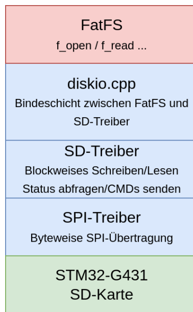
Abbildung 14: Implementierungsstack für das FatFS-Dateisystem
