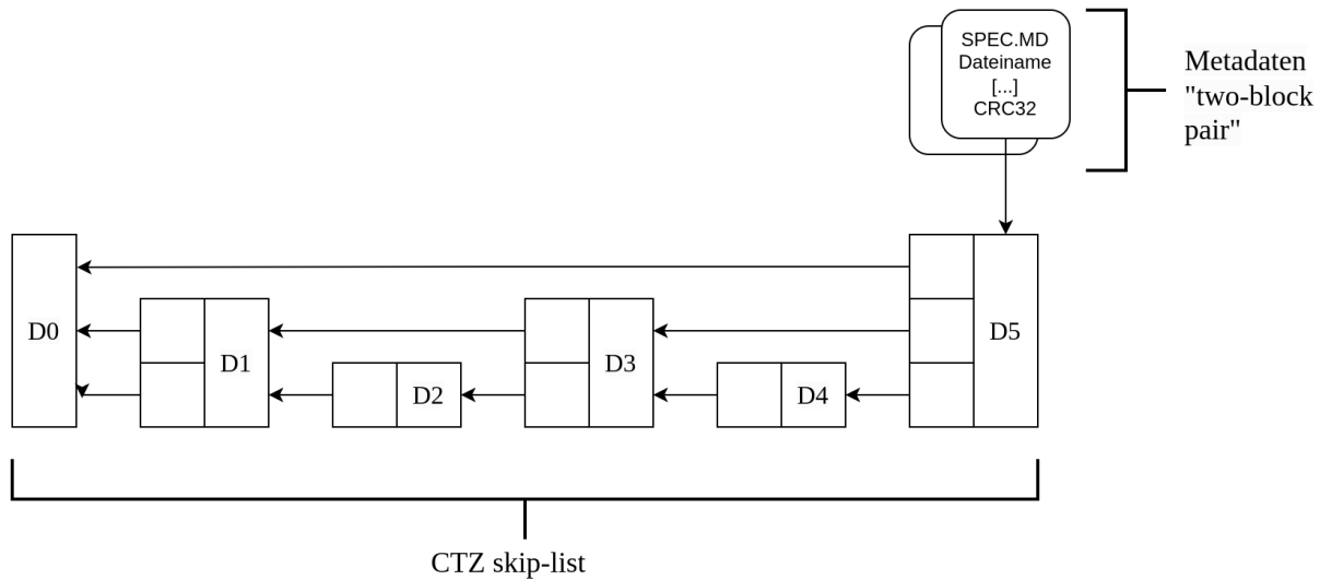
Abbildung 16: Prinzip des Dateiaufbaus bei littlefs
