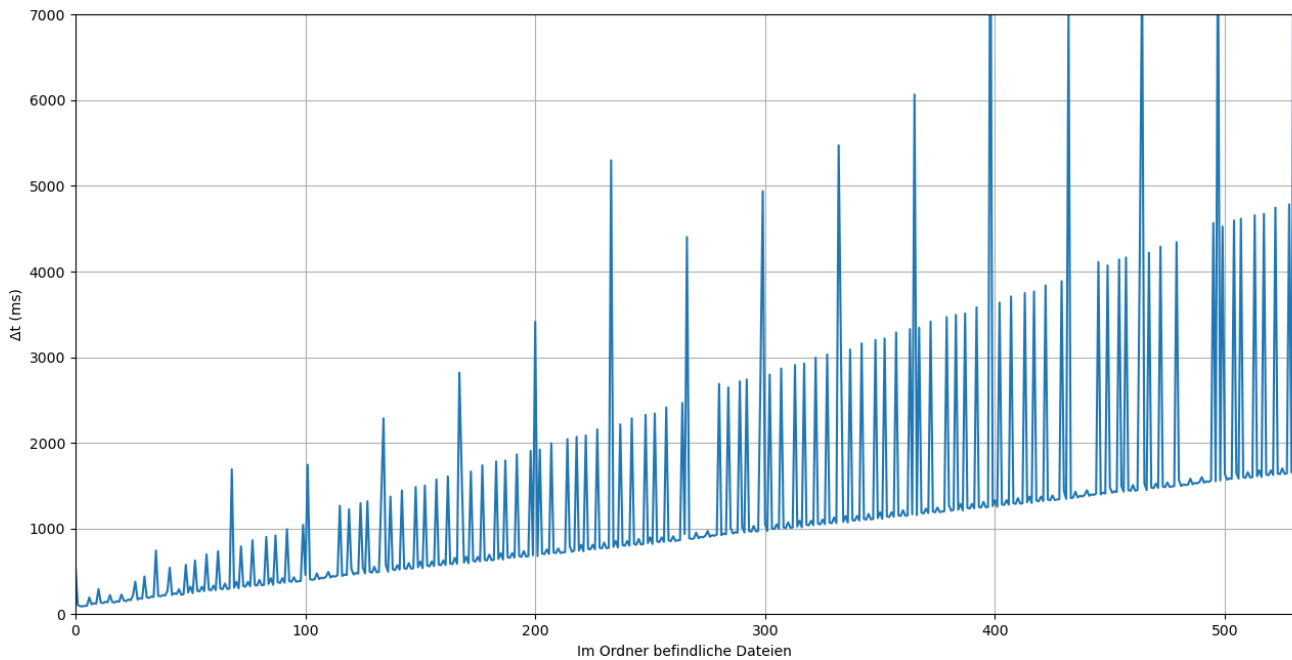
Abbildung 21: Dauer der Neuerstellung von Dateien auf dem littlefs-Dateisystem mit korrupten Daten
