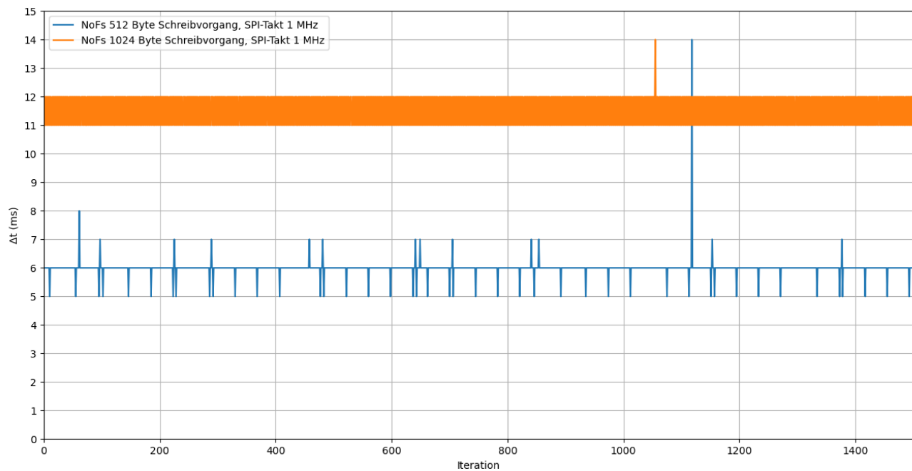
Abbildung 29: Dauer von 512 Byte und 1024 Byte Schreibvorgängen
