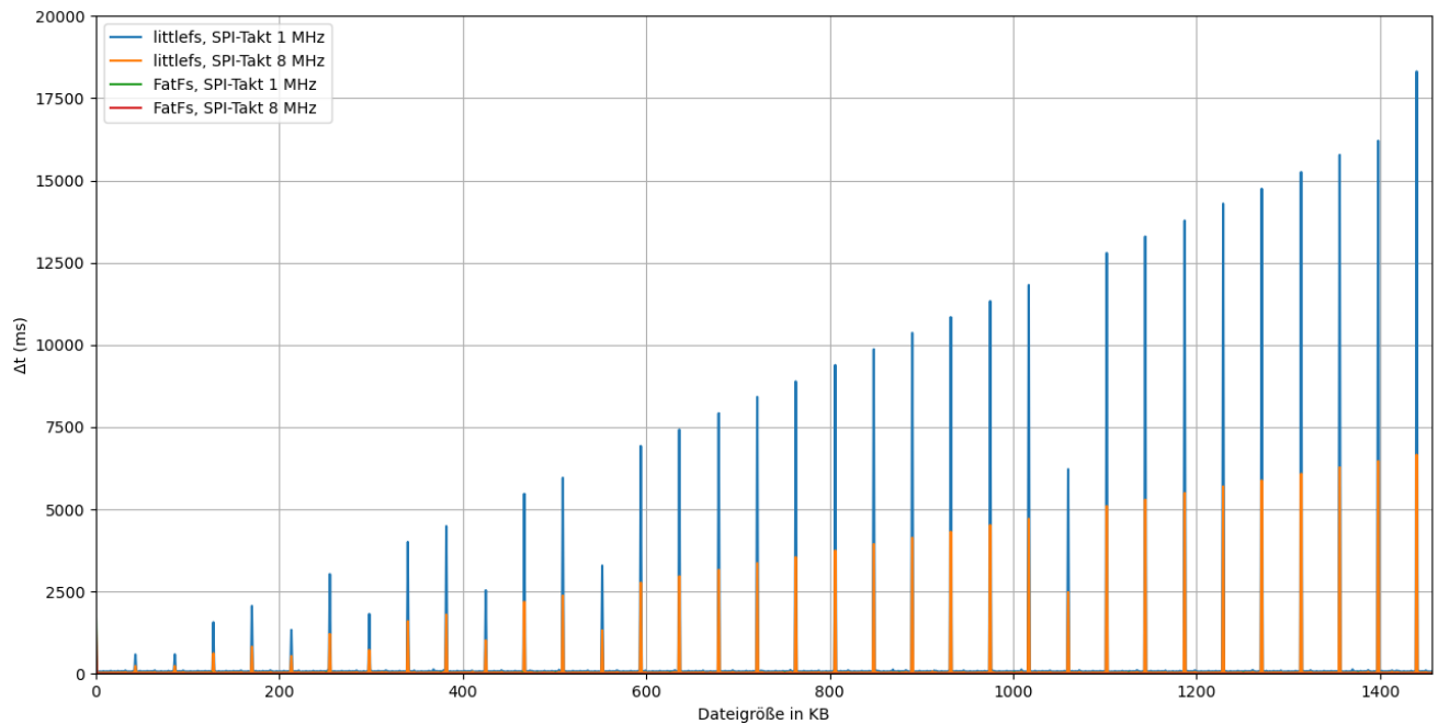
Abbildung 25: Dauer des Anhängens von 1 KB an eine Datei in Abhängigkeit der Dateigröße
