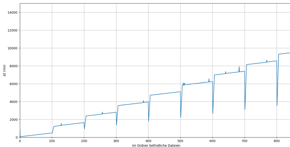
Abbildung 16: Dauer der Neuerstellung von Dateien auf dem FatFs-Dateisystem
