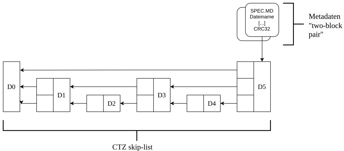
Abbildung 19: Prinzip des Dateiaufbaus bei littlefs
