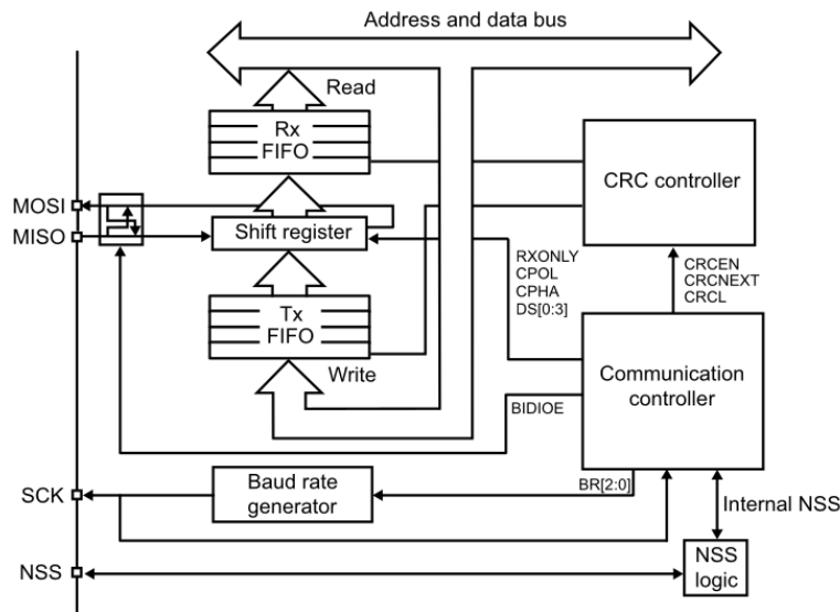
Abbildung 10: Blockdiagramm für die SPI-Peripherie des STMG431[4]
