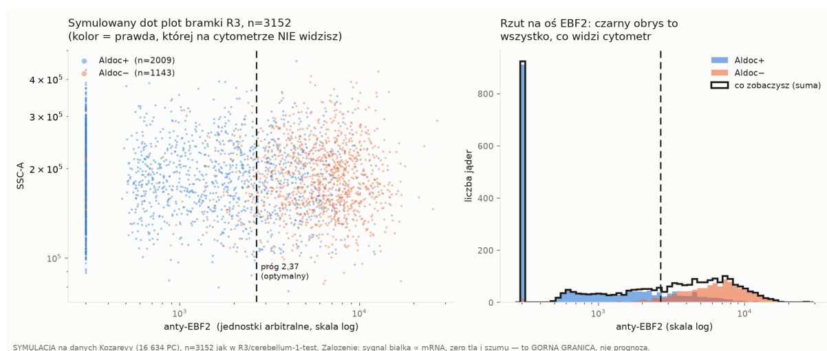
Rysunek 3.2. Symulacja wykresu punktowego dla bramki R3 przy 3 152 zdarzeniach, czyli tylu, ile było w próbce cerebellum-1-test. Kolory pokazują prawdę, której na cytometrze nie widać. Czarny obrys po prawej to wszystko, co widzi aparat. Skrypt 43_symulacja_bramki_ebf2.py.
