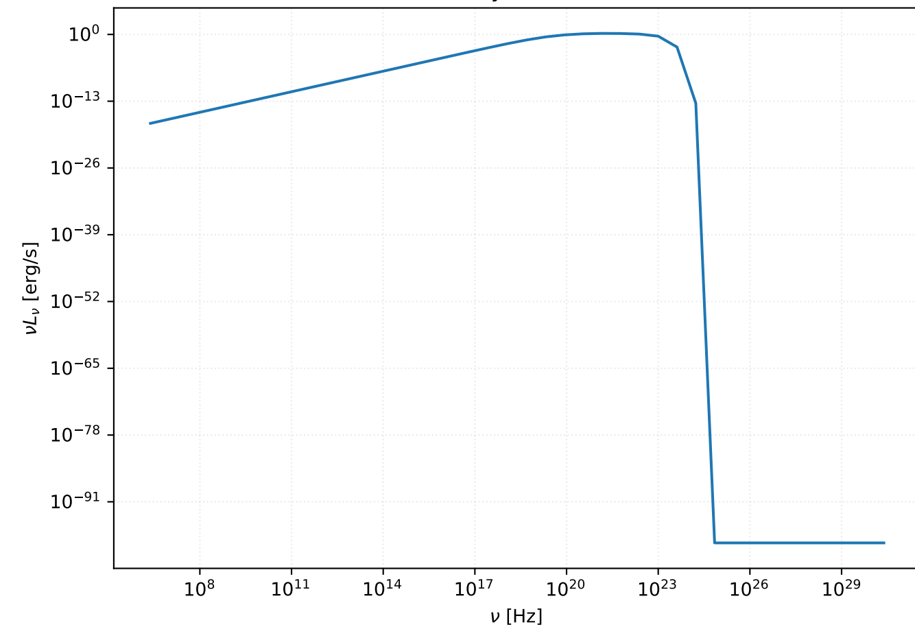
Pion IC
