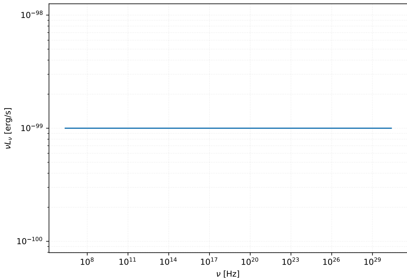
Muon IC
