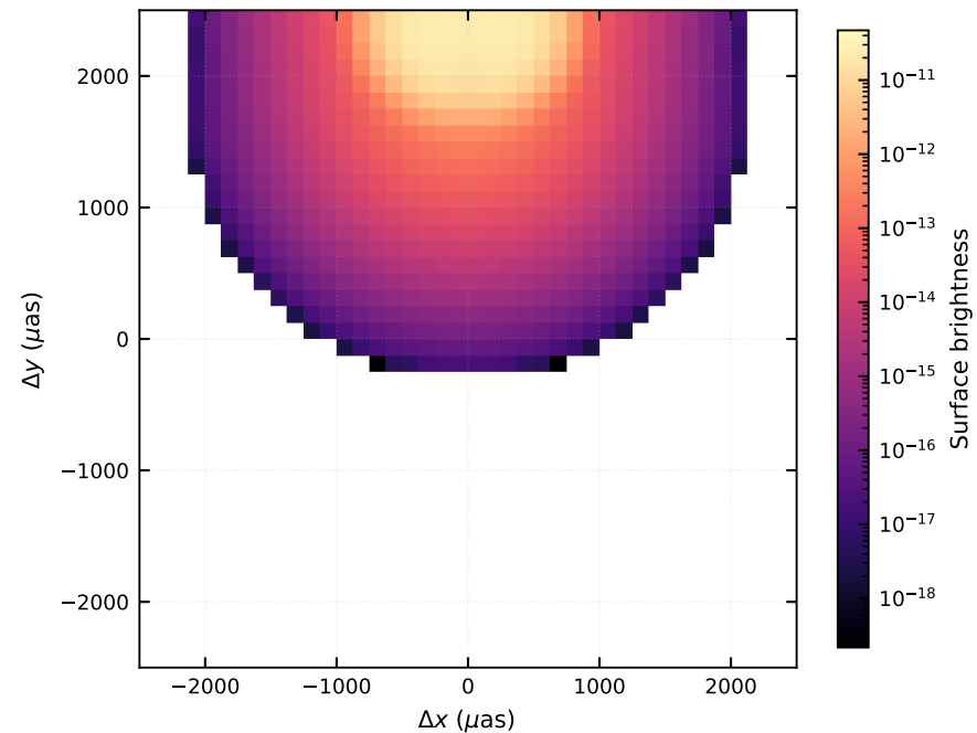
VegasAfterglow, 1.0e+08 s
