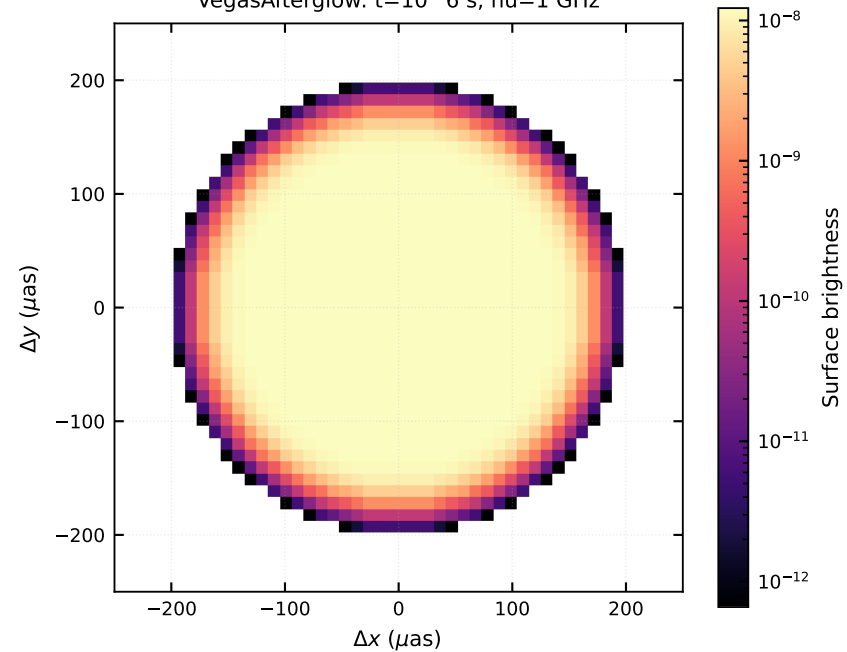
VegasAfterglow: t=10^6 s, \nu=1 GHz
