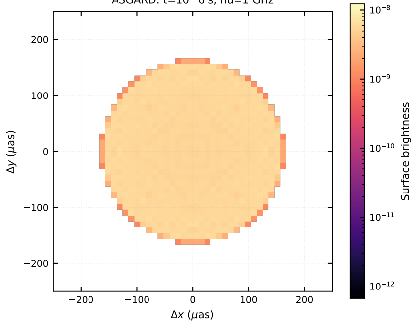
ASGARD: t=10^6 s, \nu=1 GHz
