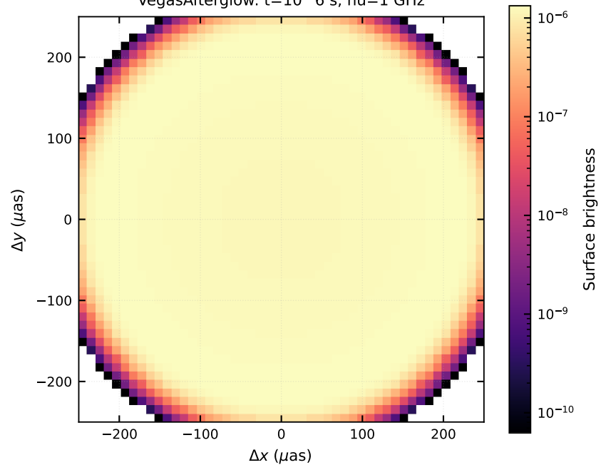
VegasAfterglow: t=10^6 s, \nu=1 GHz
