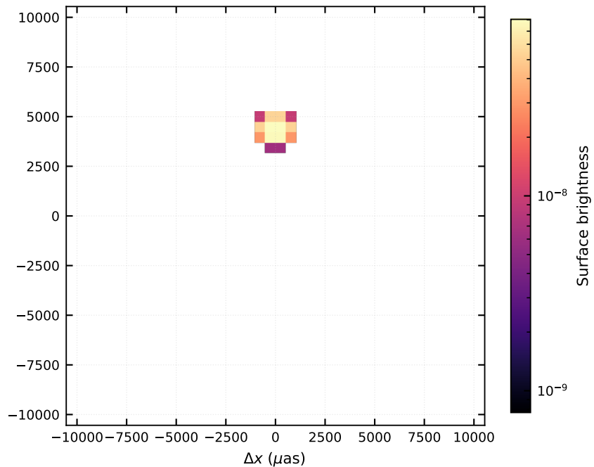
VegasAfterglow, 1.0e+08 s
