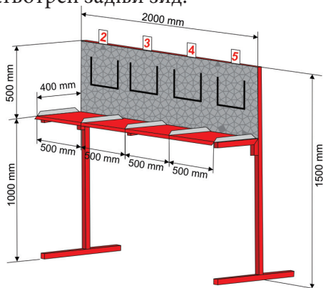
Слика 11. Постоље за постављање ватрогасних арматура
