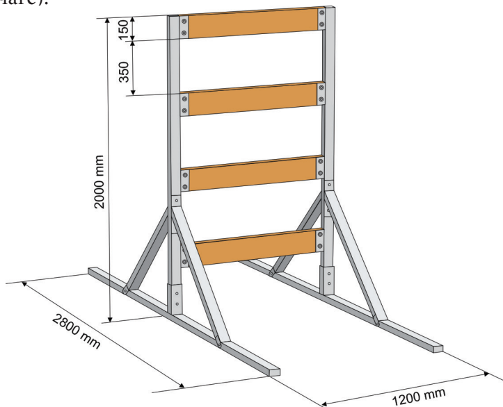
Слика 28. Широка лества
