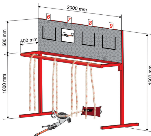
Слика 10. Постоље са гредом
