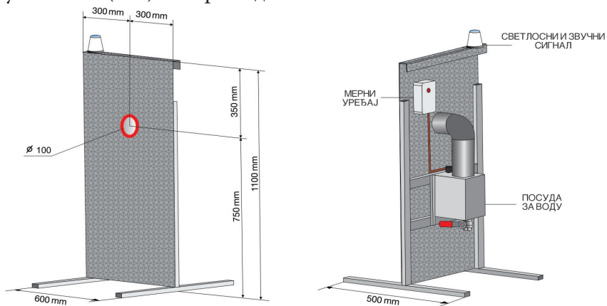
Слика 9. Зид за уливање воде
